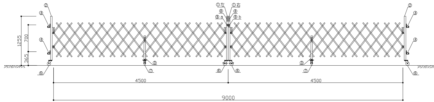
正面図
