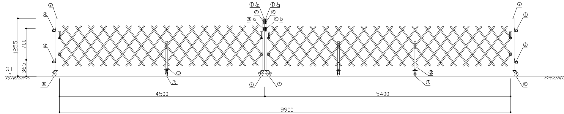
正面図
