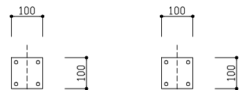
⑦キャスター-100φシングル詳細
