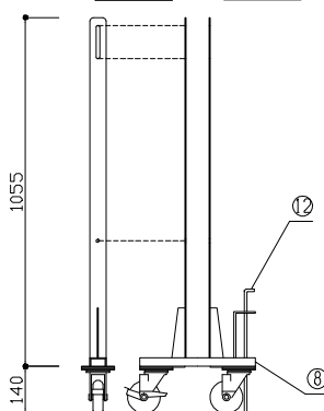
⑤中間脚詳細
