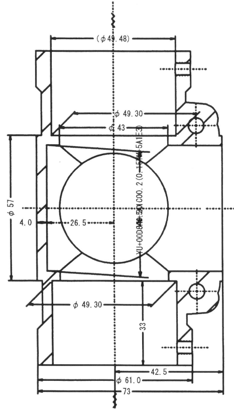
A-A 断面図
