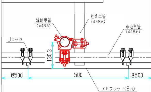
あ部分 取付詳細図
