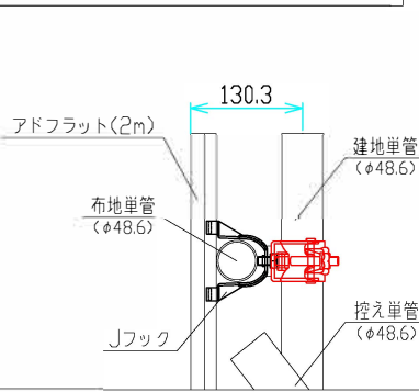
い部分 取付詳細図
