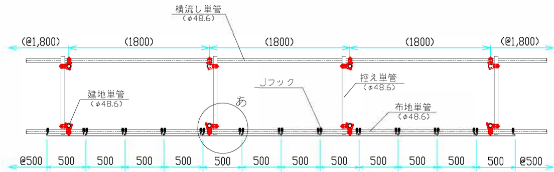
平面図
