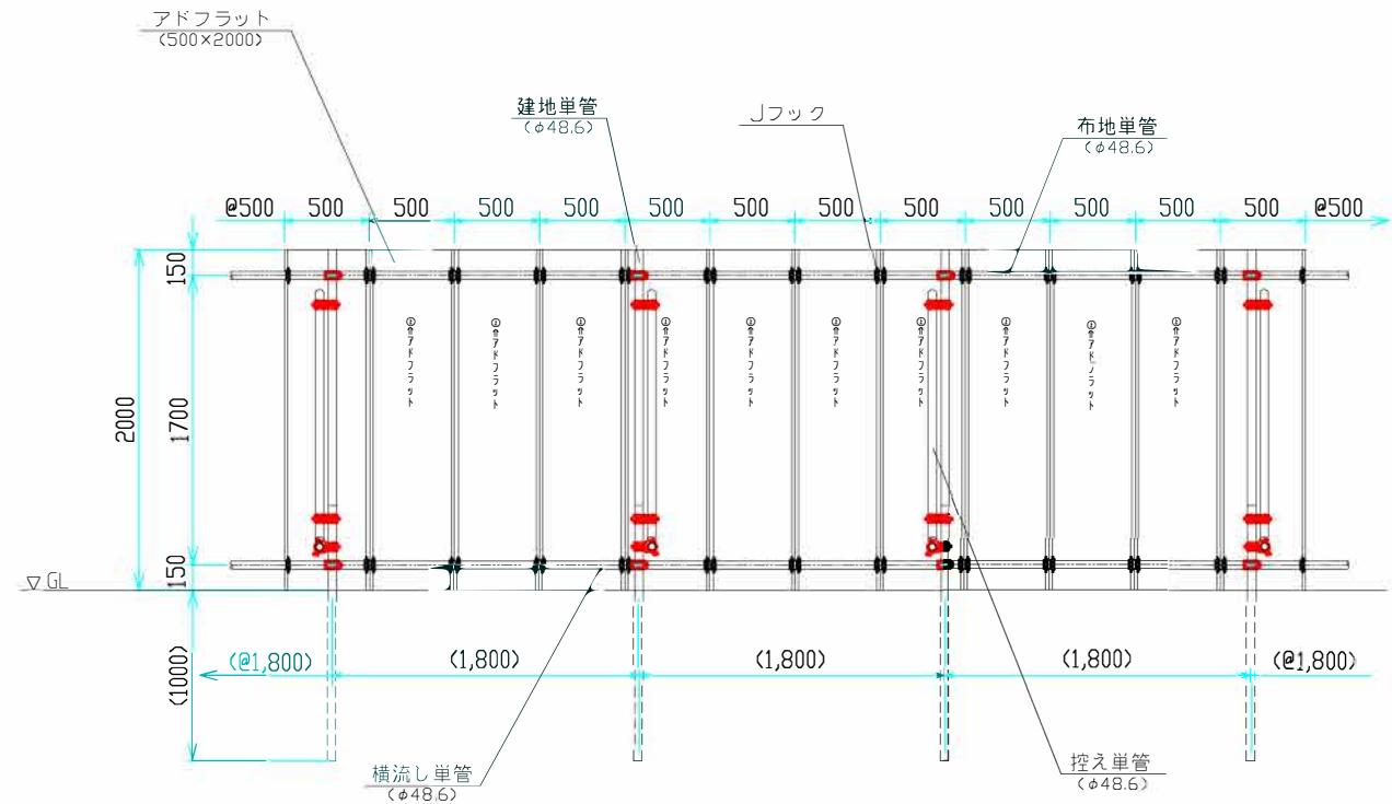
立面図
