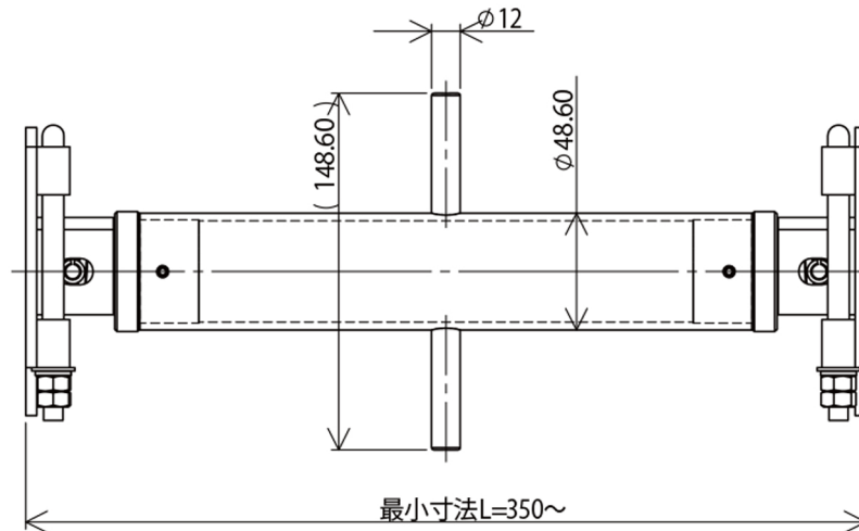
両ネジタイプ (25-38 型以外)
