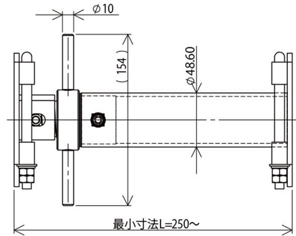
片ネジタイプ (25-38型)
