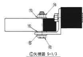
③矢視図 S=1/3
