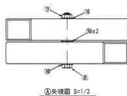
①矢視図 S=1/3
