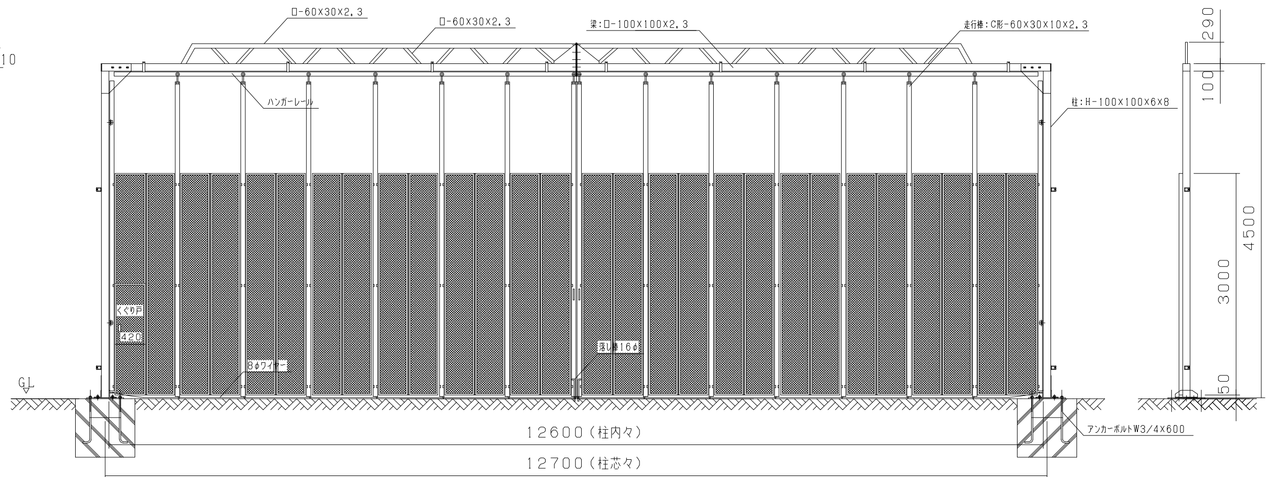
側面図
