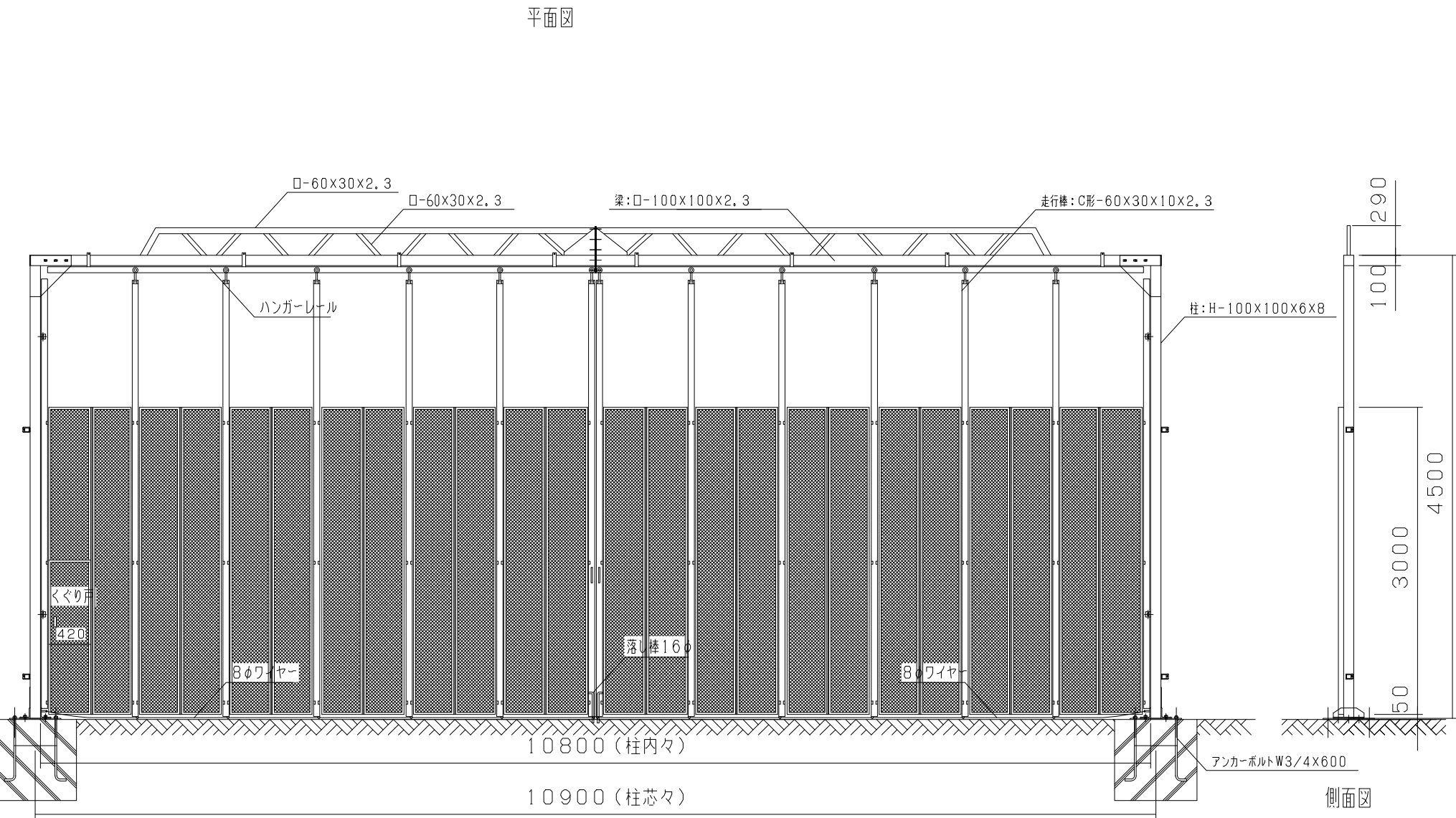
立面図
