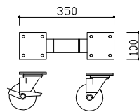
⑦キャスター100φ(ダブル)詳細図
