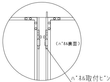
(A) ハネ取付部詳細
