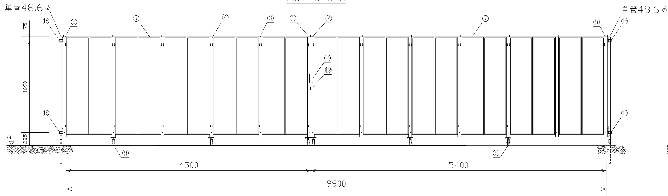
正面図 S=1/40
