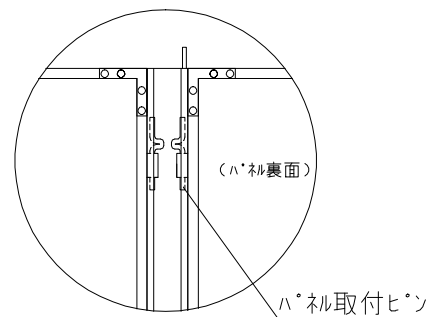
(A) ハネ取付部詳細
