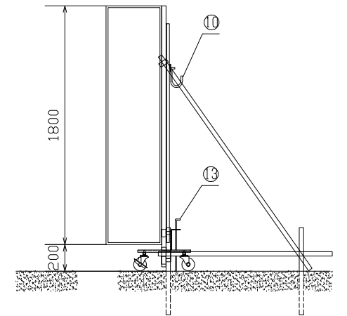
⑨キャスター台詳細図
