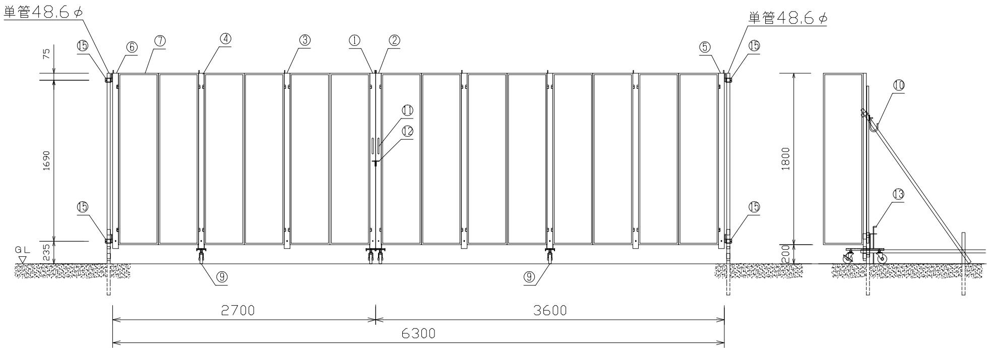
正面図 S=1/40
