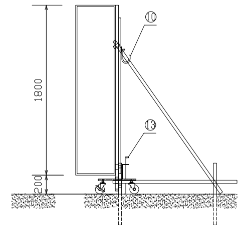
⑨キャスター台詳細図
