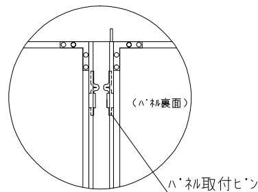
(A) ハネル取付部詳細
