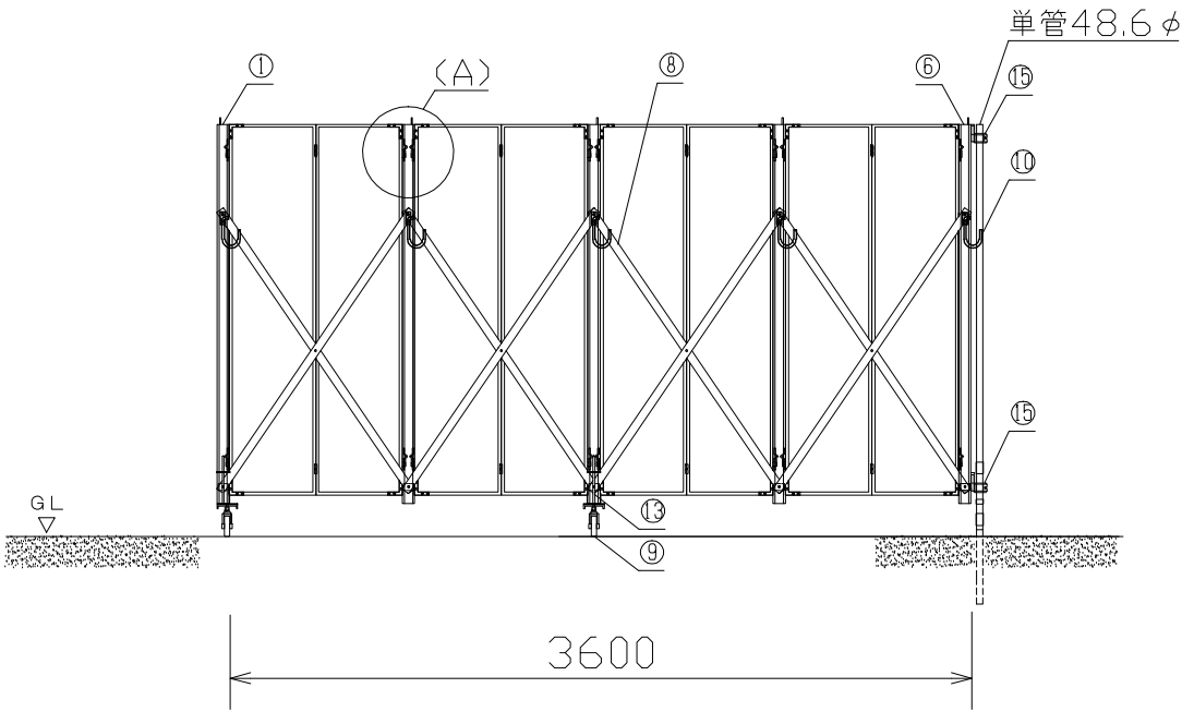
SRG-9 部材表
