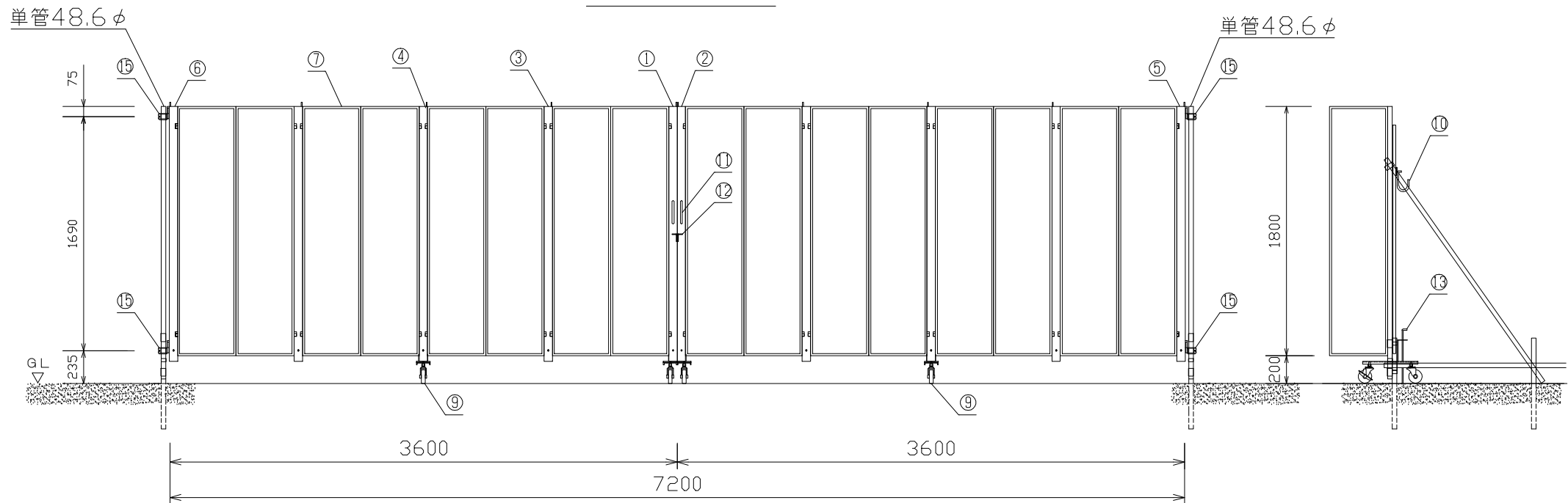
正面図 S=1/40
