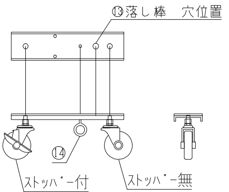
⑨キャスター台詳細図
