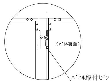
(A) ハンドル取付部詳細
