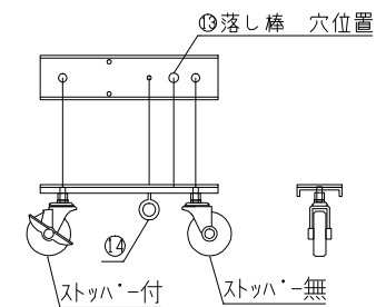
⑨キャスター台詳細図
