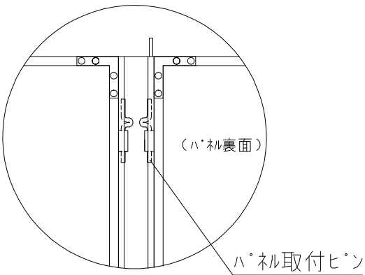
(A) ハネ取付部詳細
