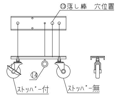
⑨キャスター台詳細図
