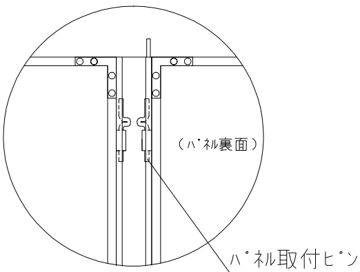
(A) ハ・ル取付部詳細
