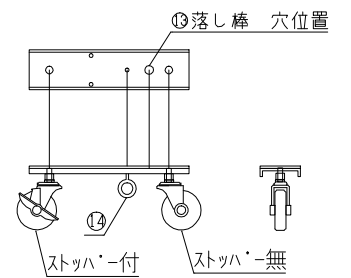
⑨キャスター台詳細図
