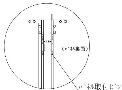
(A) ハ・ル取付部詳細
