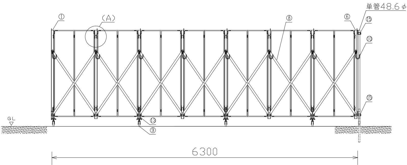
背面図 S=1/40
