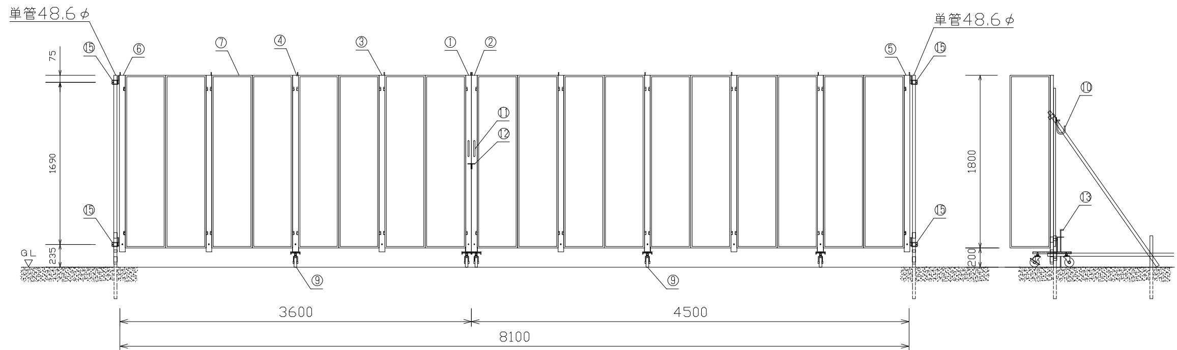
正面図 S=1/40
