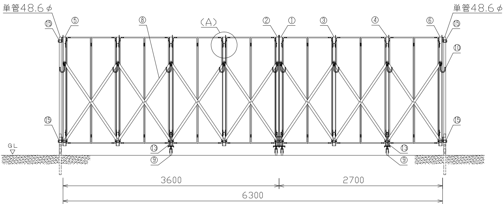
SRG-9 部材表
