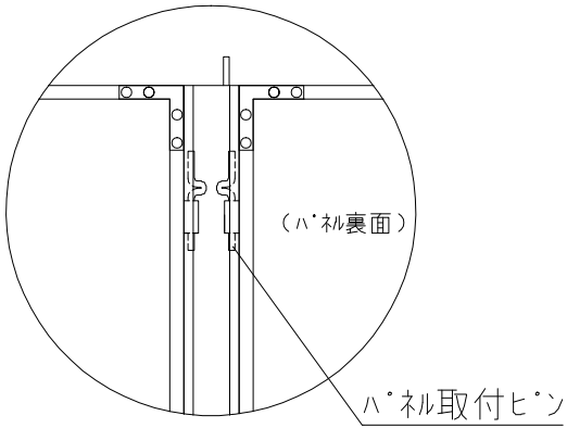
(A) ハール取付部詳細
