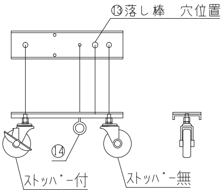
⑨キャスター台詳細図
