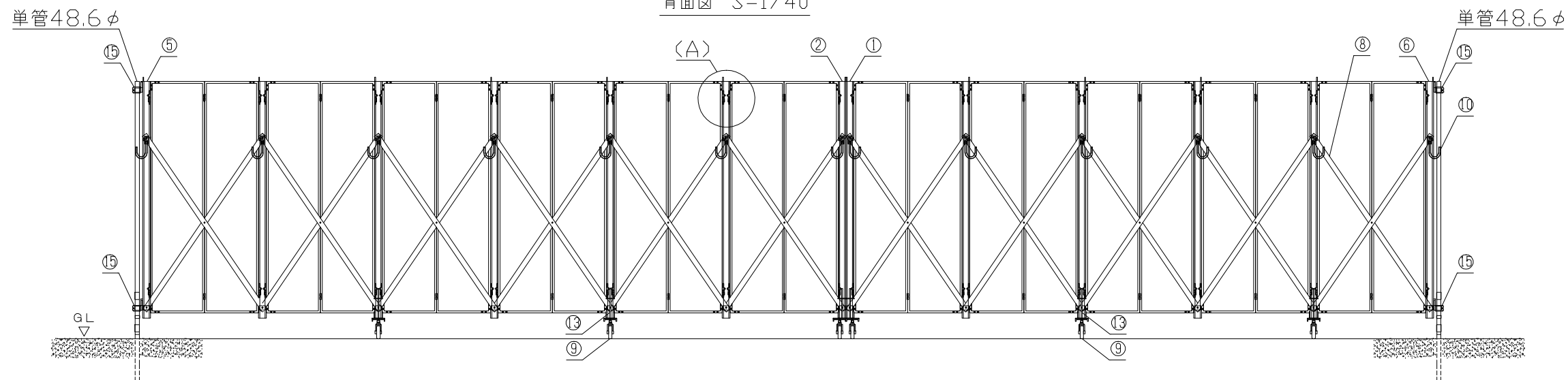
背面図 S=1/40
