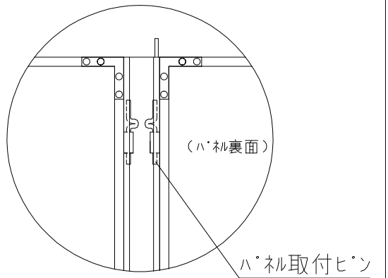
(A) ハネ取付部詳細
