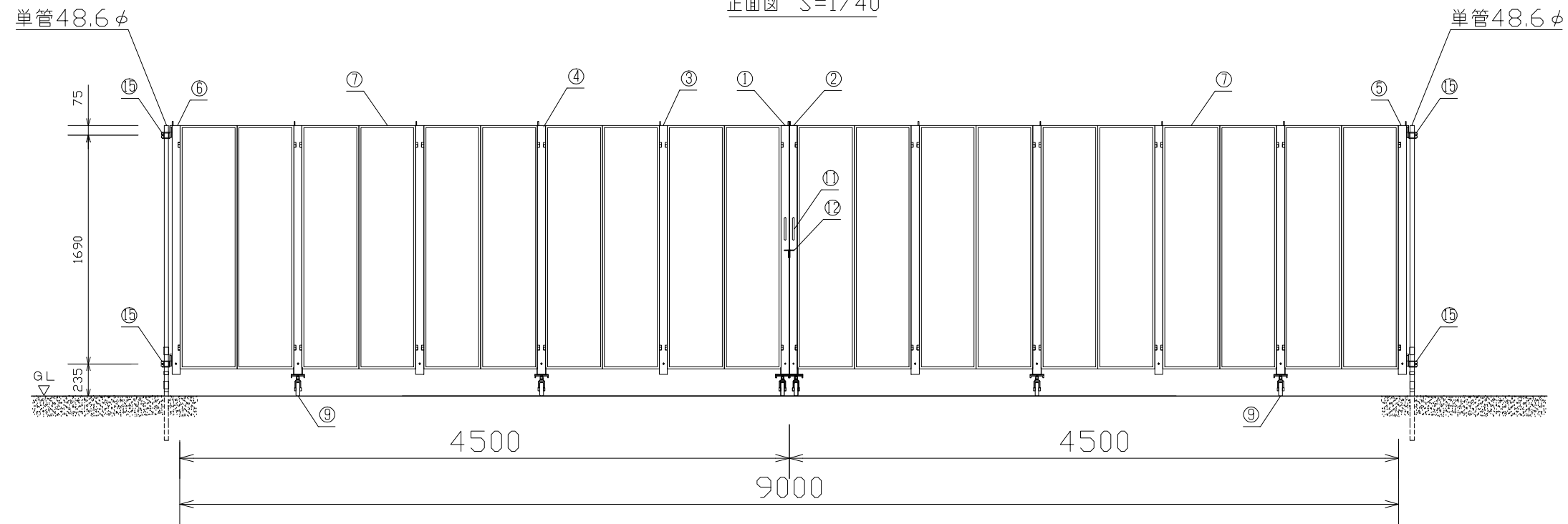
正面図 S=1/40
