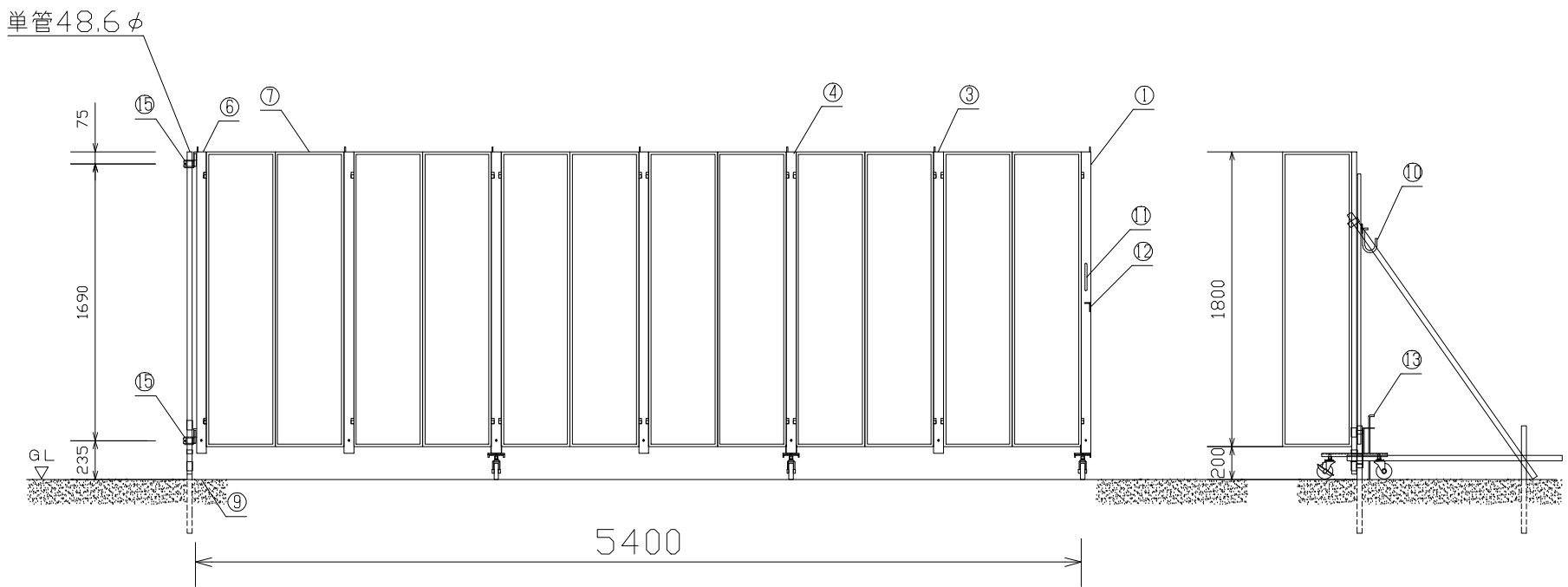
正面図 S=1/40
