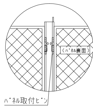
(A) ハネ取付部詳細
