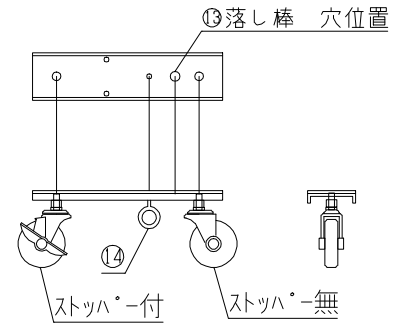
⑨キャスター台詳細図
