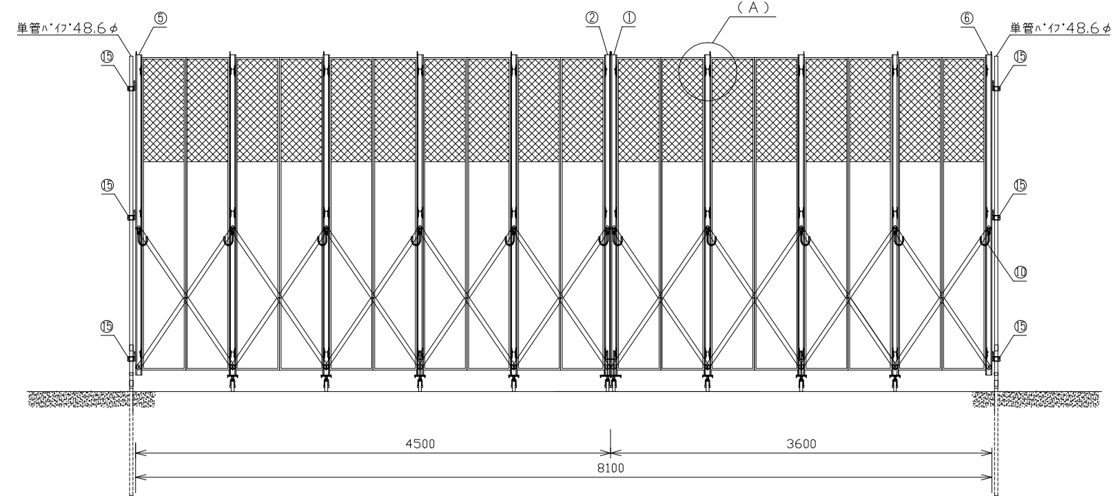
背面図 S=1/50
