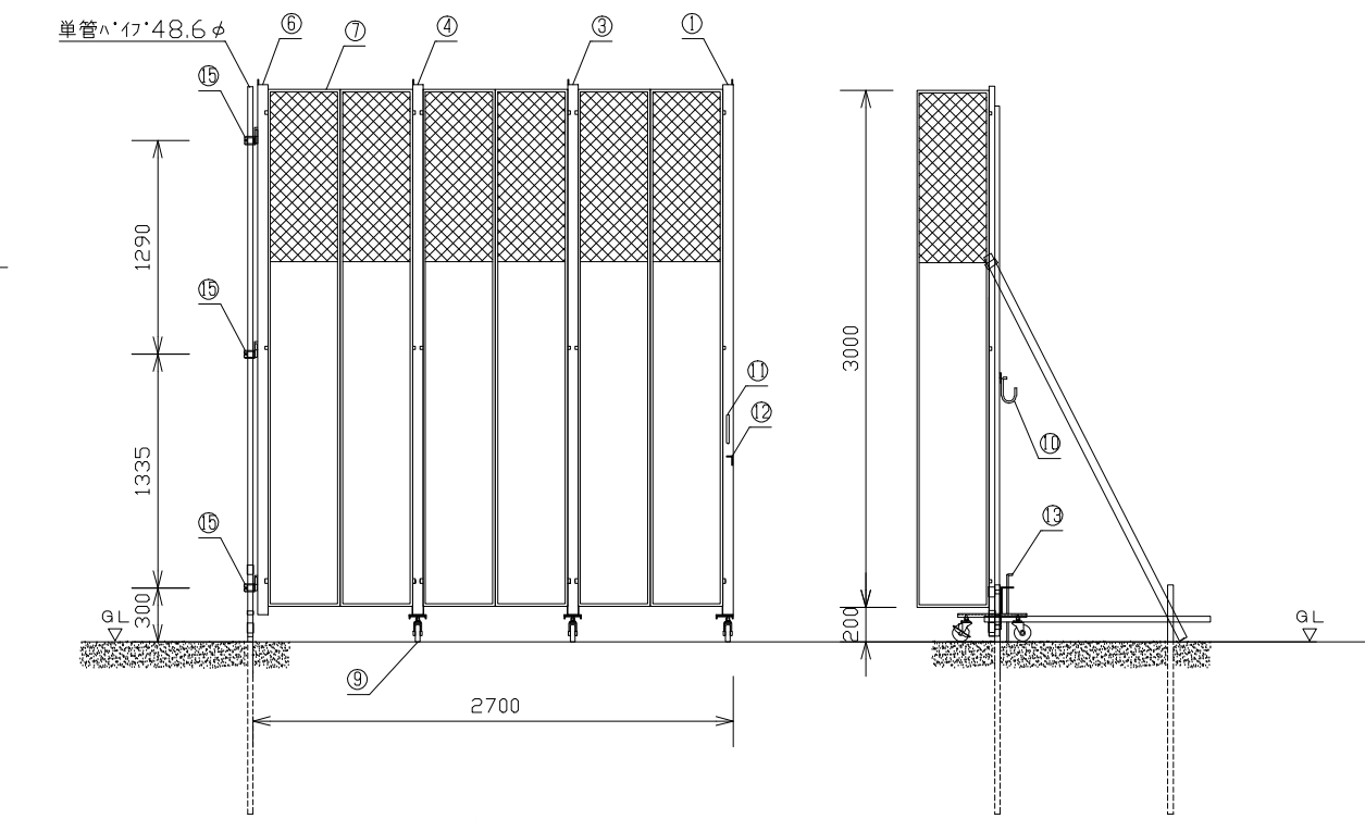
正面図 S=1/50
