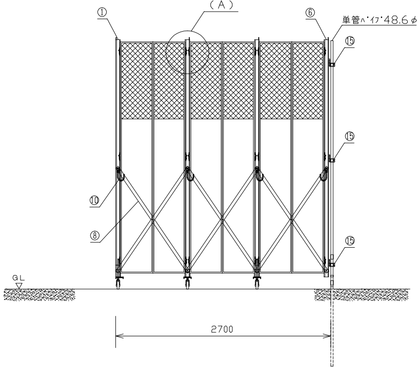
背面図 S=1/50
