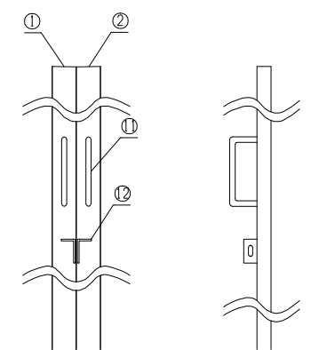
①②詳細図
