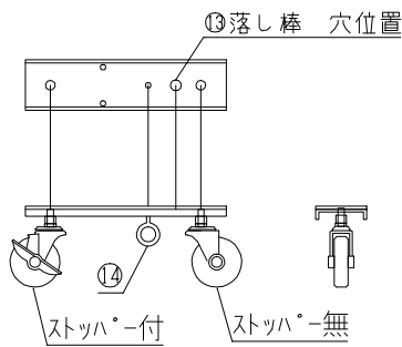
⑨キャスター台詳細図
