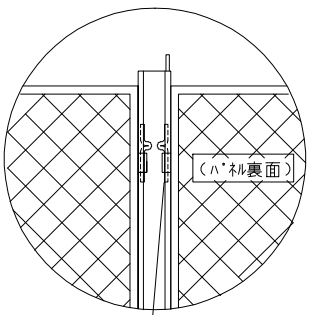
(A) ハネ取付部詳細
