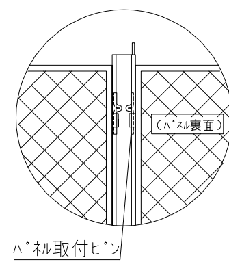
(A) ハネ取付部詳細
