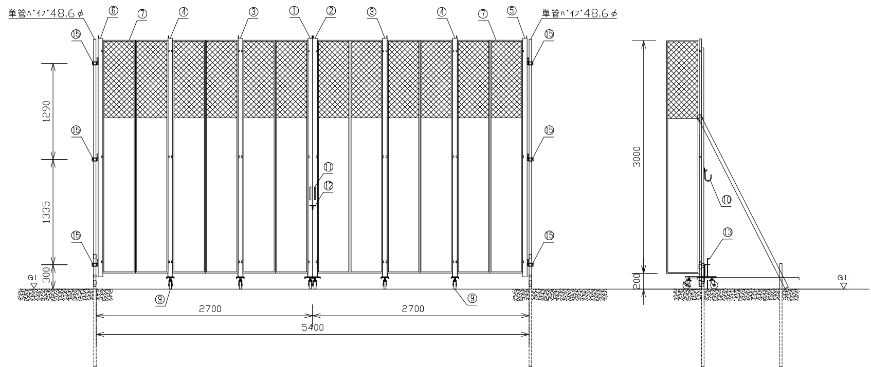
正面図 S=1/50
