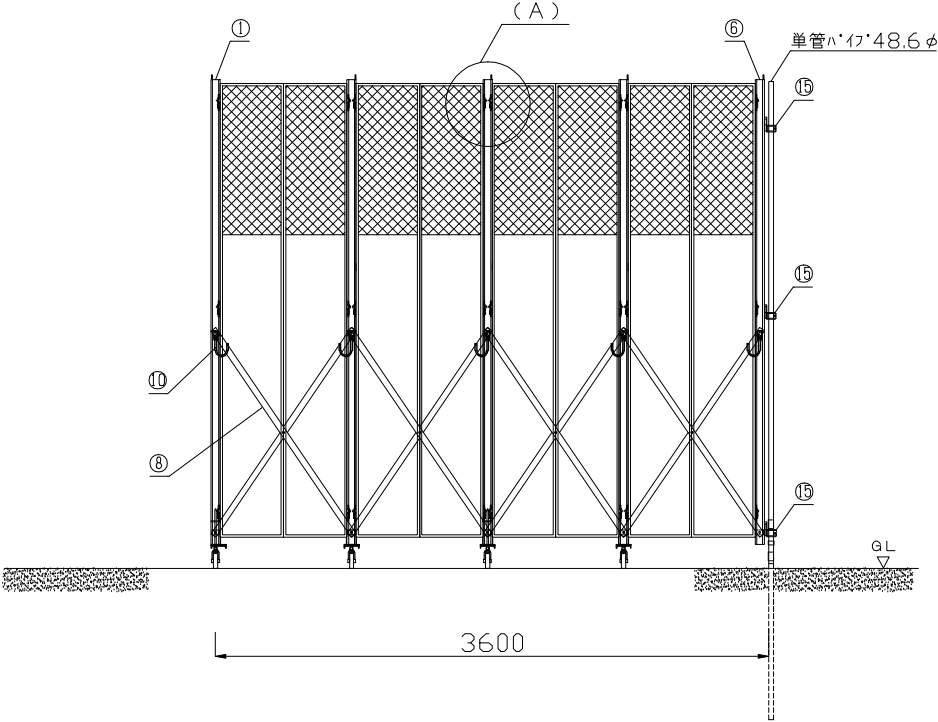
SRG-9(H3.0) 部材表
