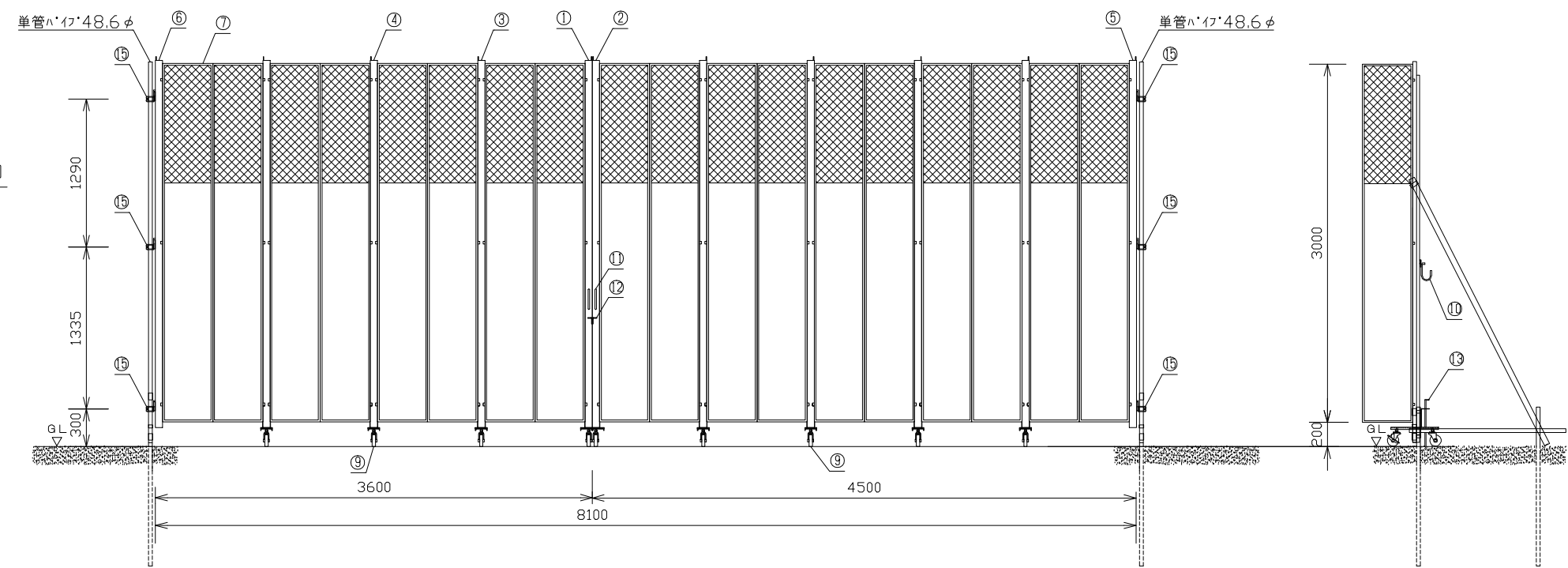
正面図 S=1/50
