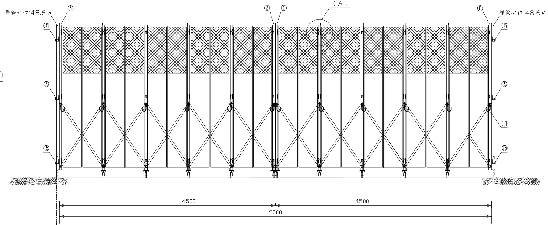
SRG-9(H3.0) 部材表
