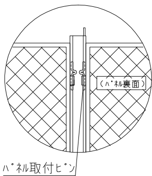
(A) ハネル取付部詳細
