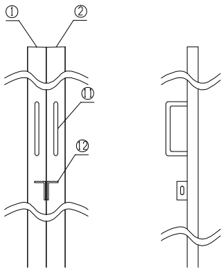
①②詳細図
