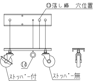
⑨キャスター台詳細図
