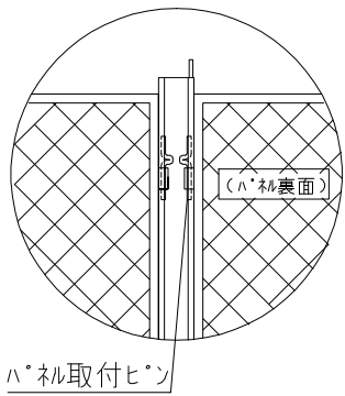
(A) ハネル取付部詳細
