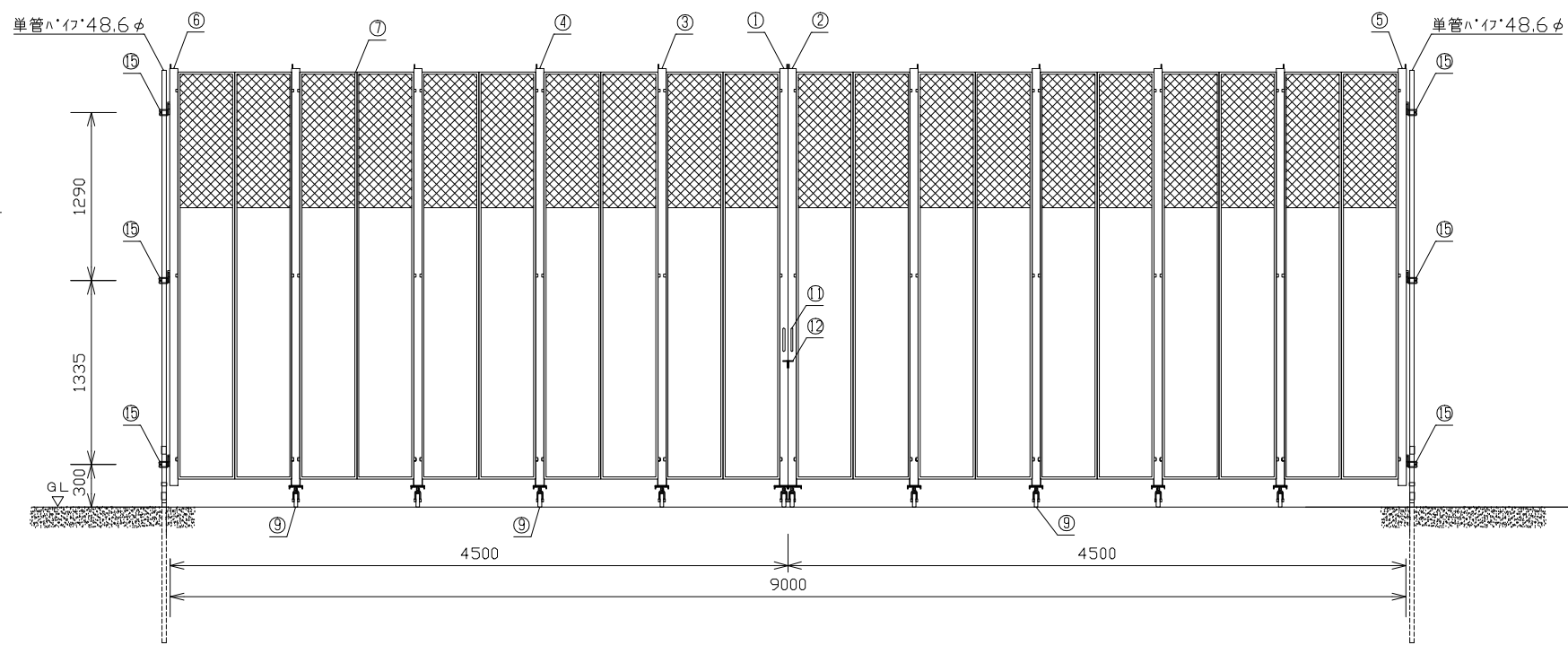
正面図 S=1/50
