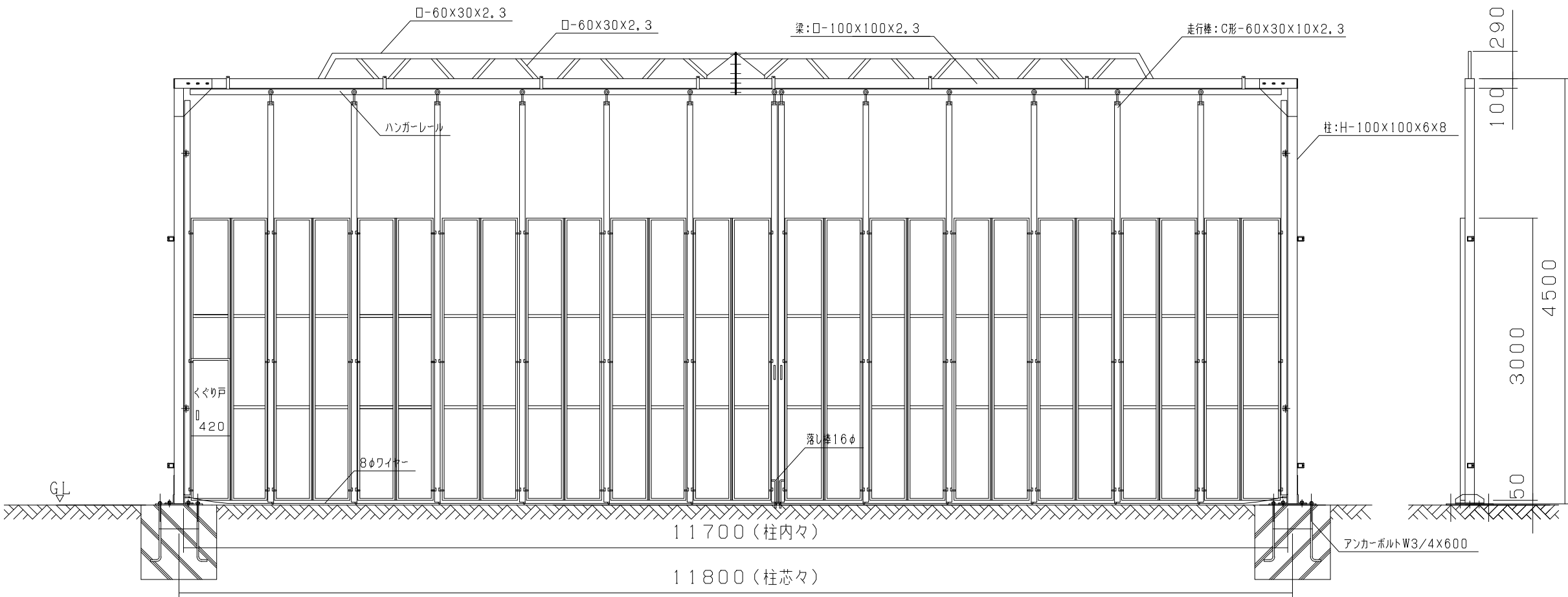
側面図
