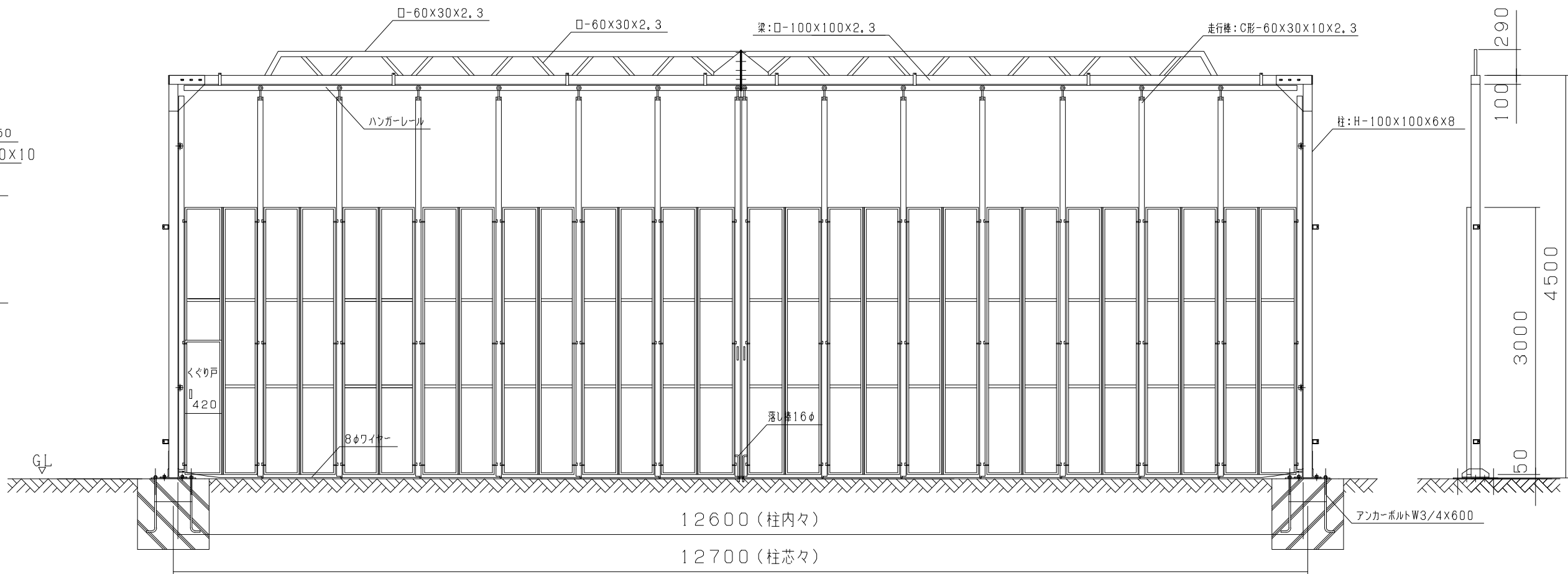
側面図
