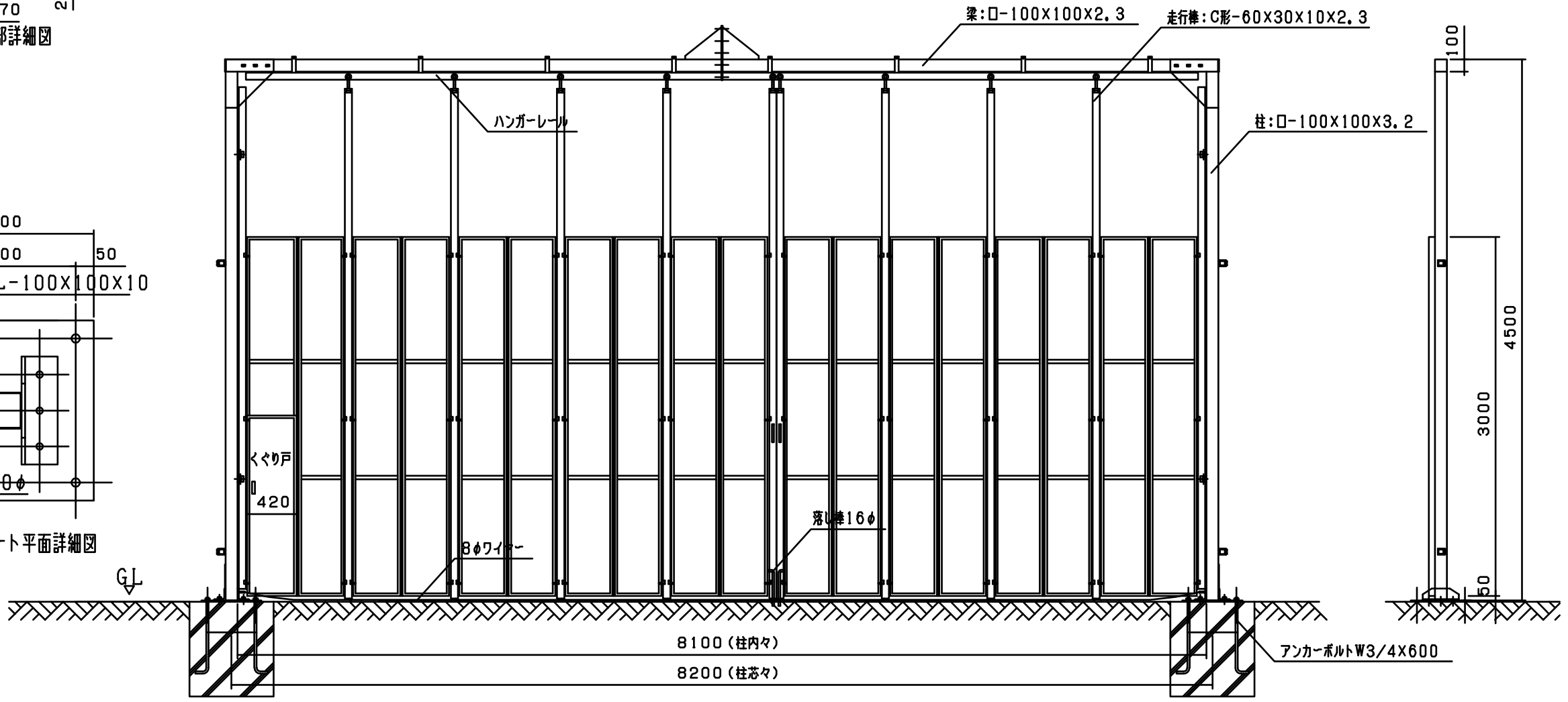
側面図
