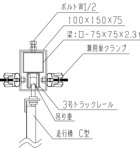
B：柱梁調整金具詳細図
