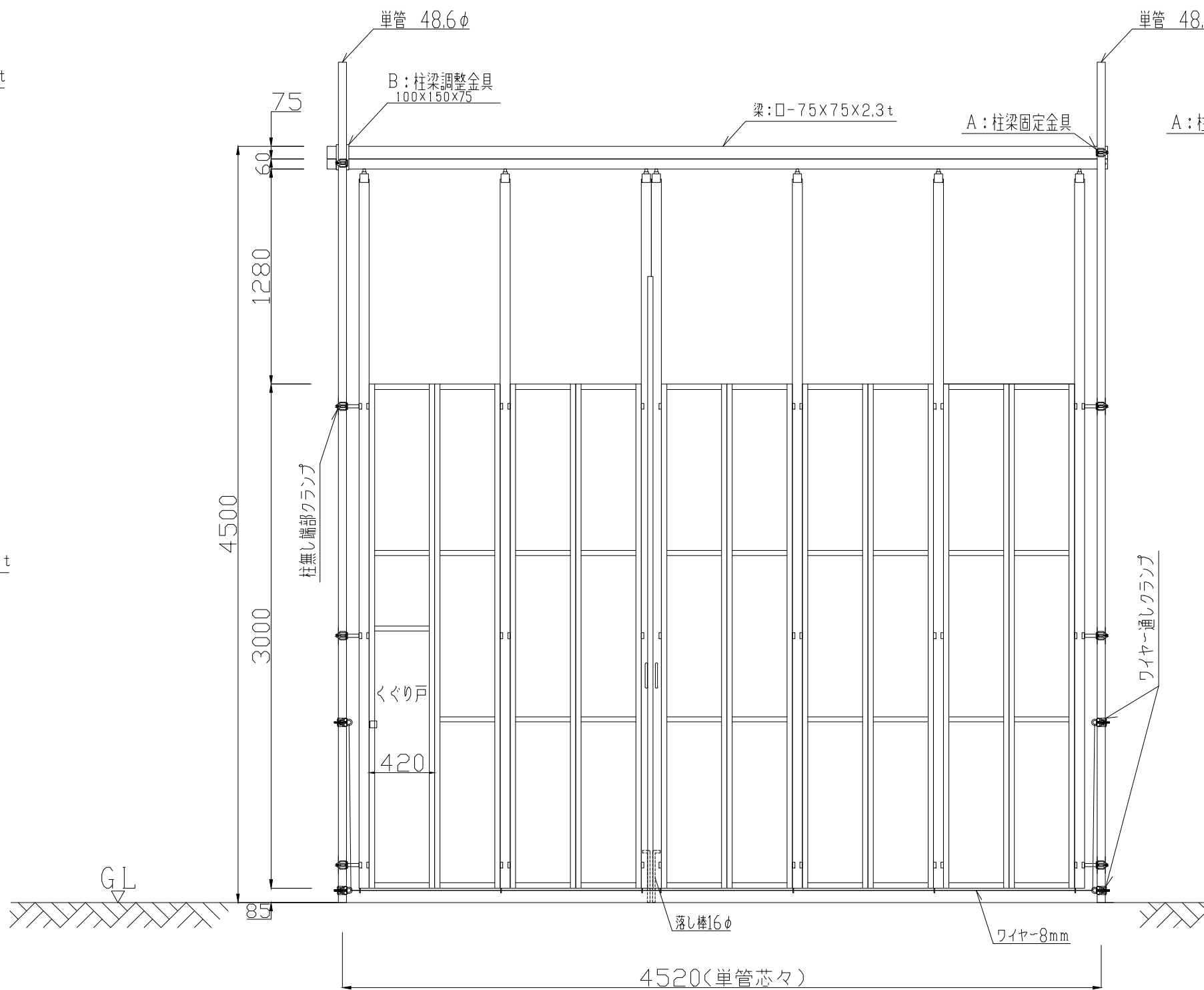
立面図
