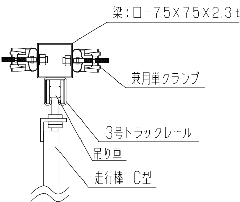
A：柱梁固定金具
