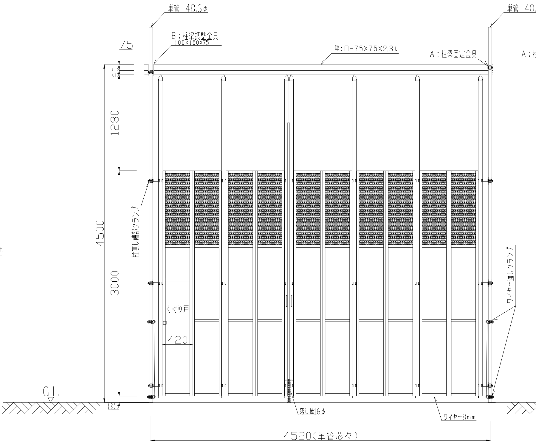
立面図
