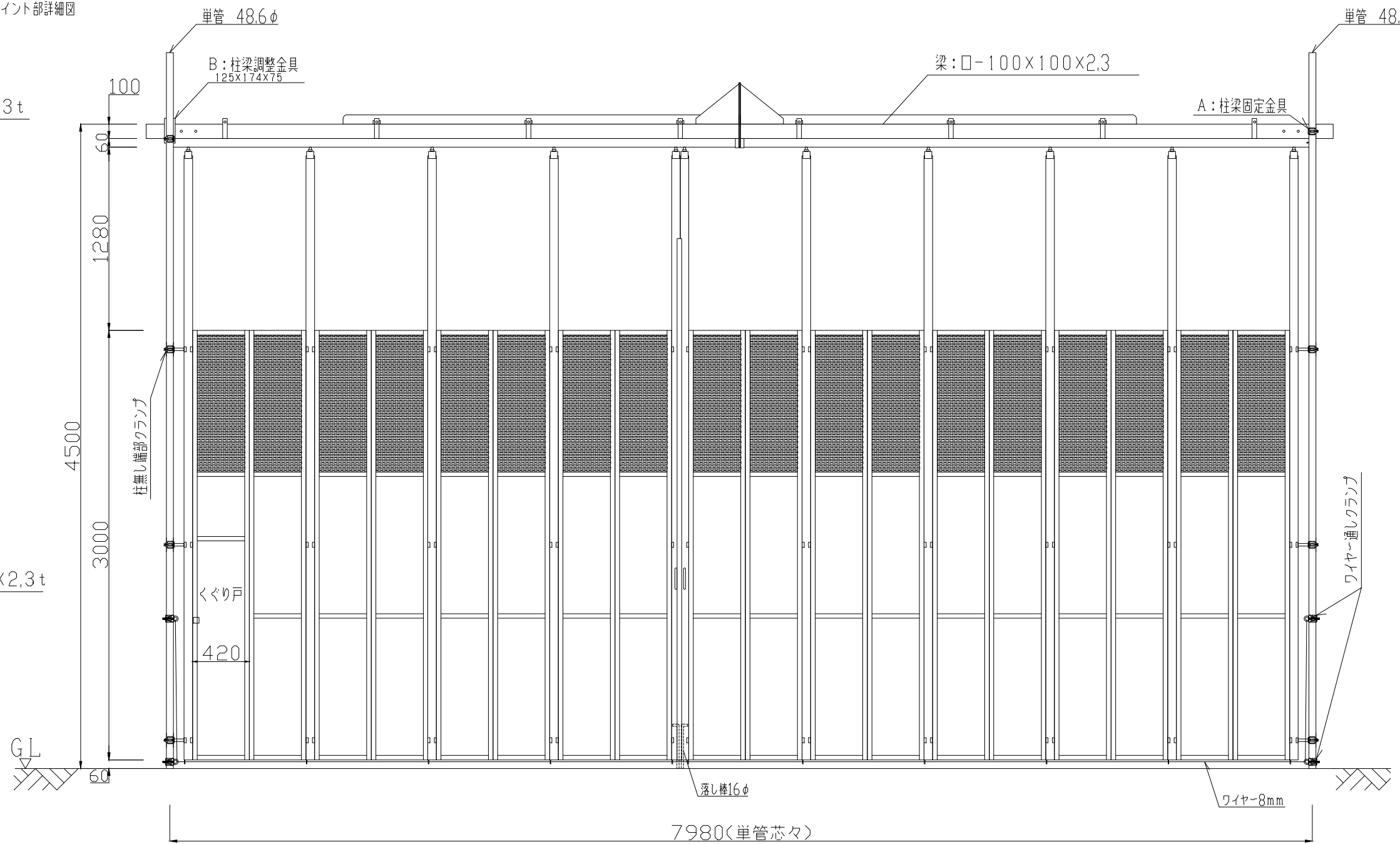
立面图
