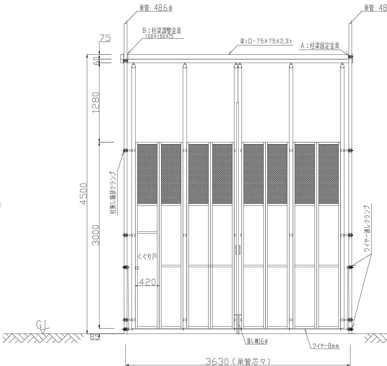
立面図
