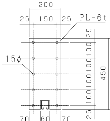
梁ジョイント部詳細図
