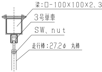
ハンガーレール断面詳細図
