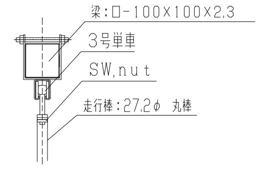
ハンガーレール断面詳細図
