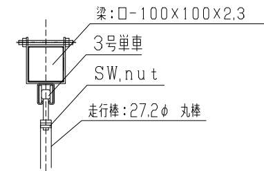
ハンガーレール断面詳細図
