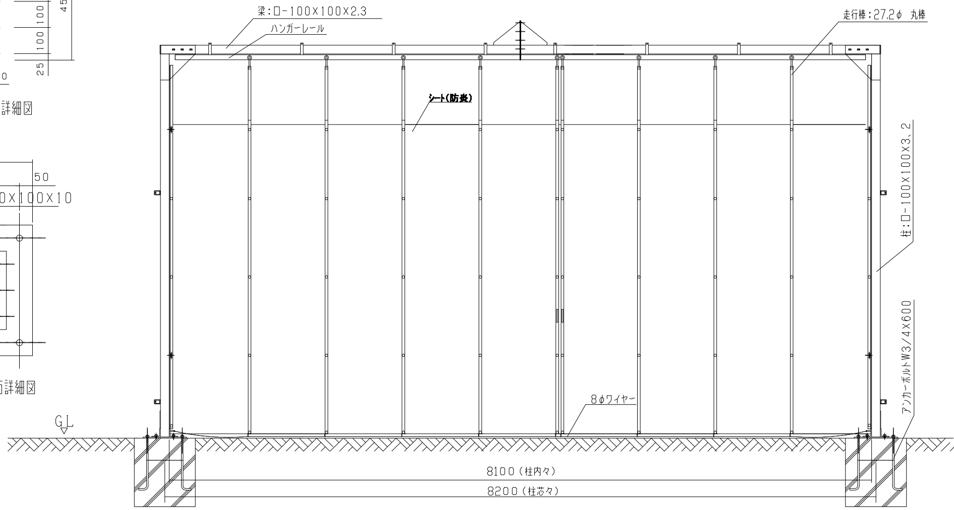
立面図
