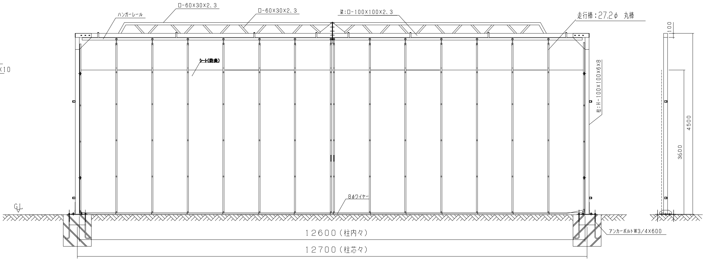
側面図
