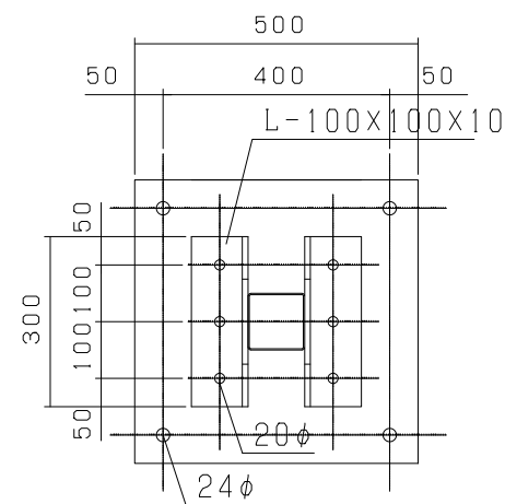
ベースプレート平面詳細図
