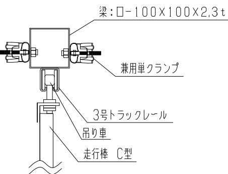
B：柱梁調整金具詳細図
