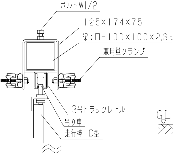
B：柱梁調整金具詳細図
