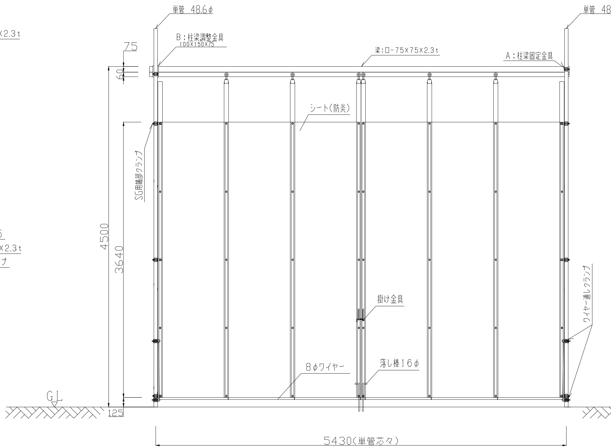
立面図
