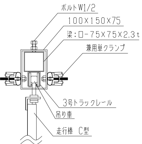
B：柱梁調整金具詳細図
