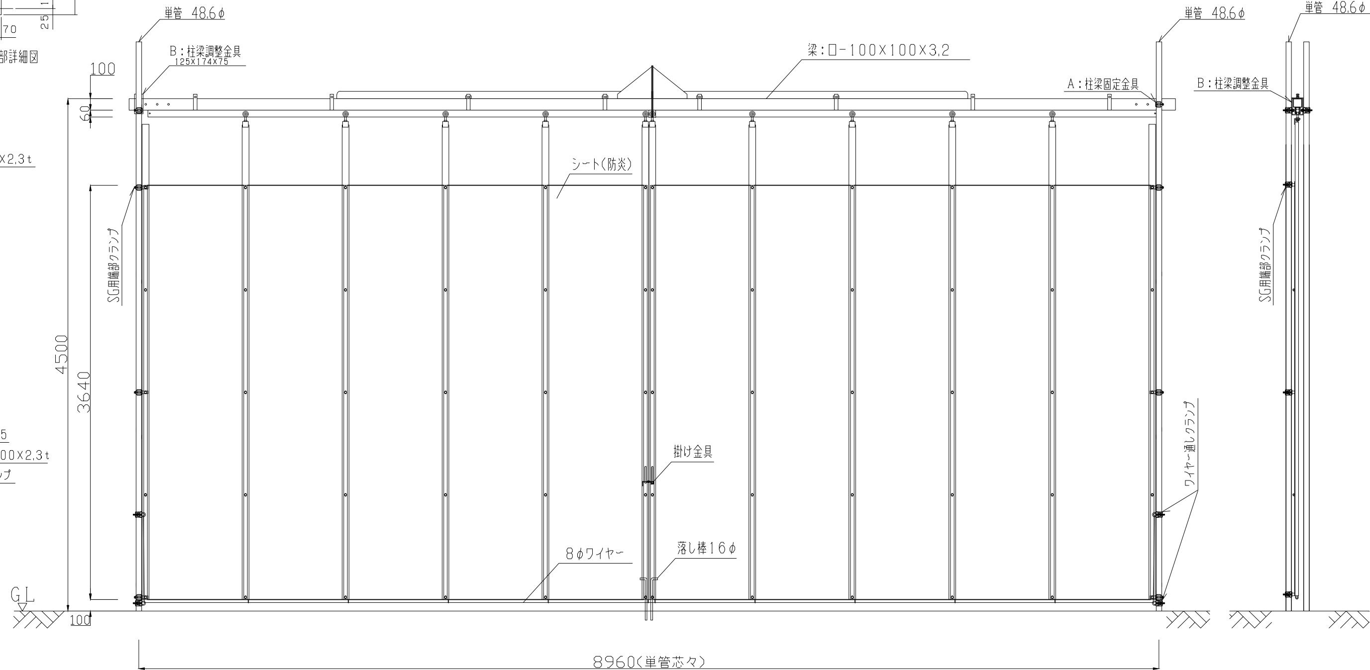
側面図
