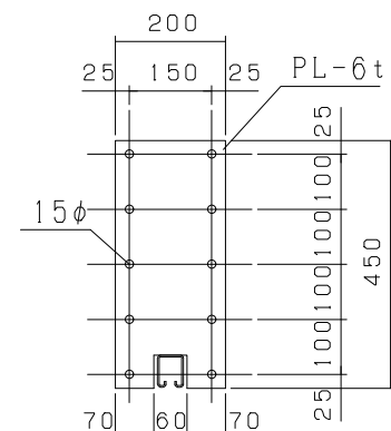
梁ジョイント部詳細図
