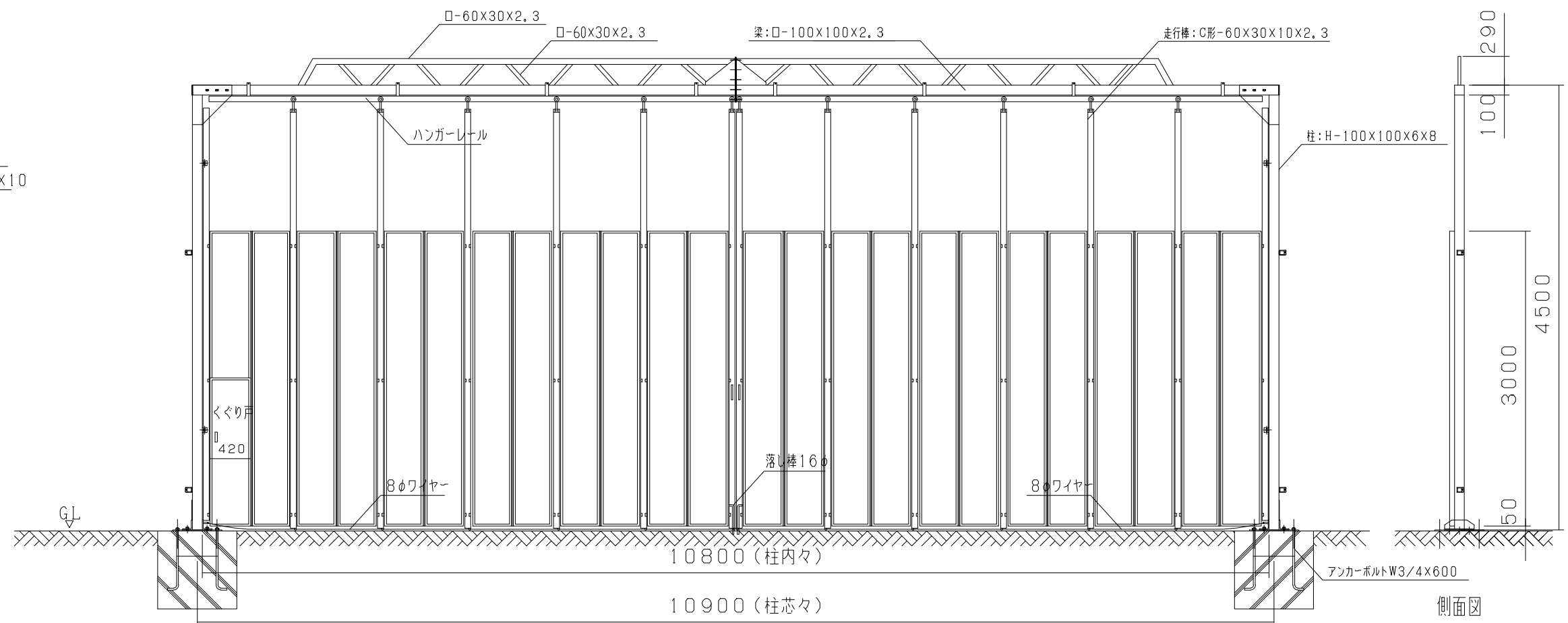
立面图
