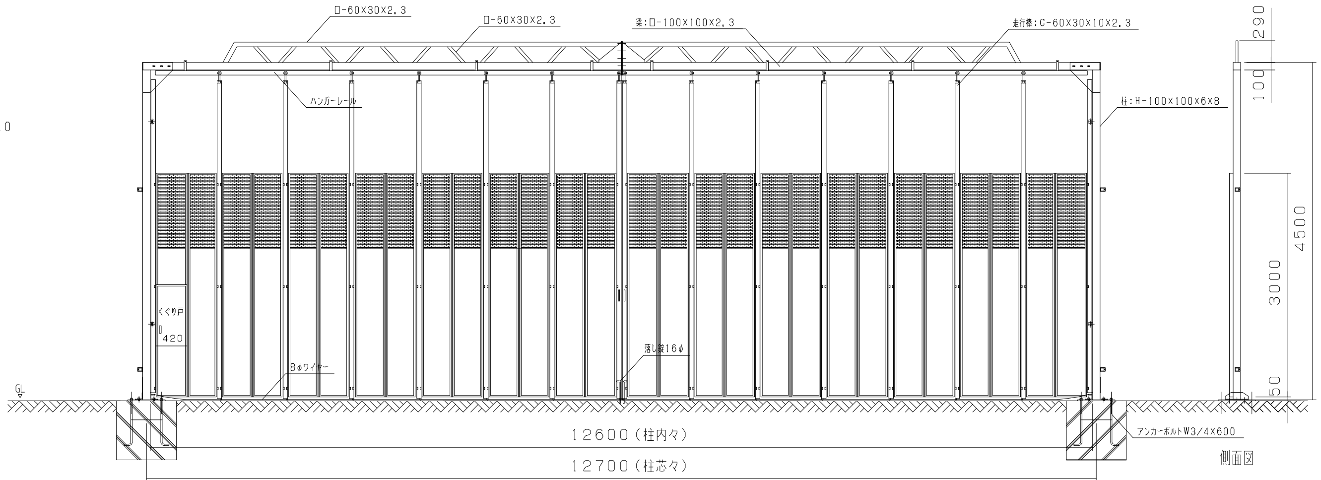
立面图
