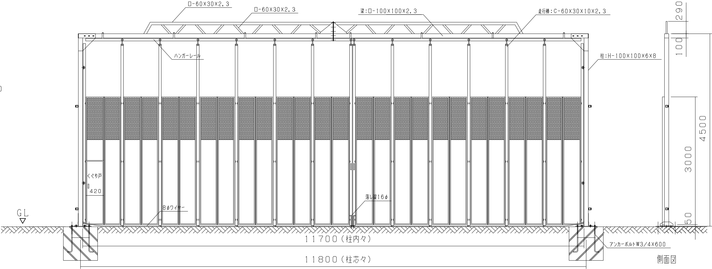
立面図
