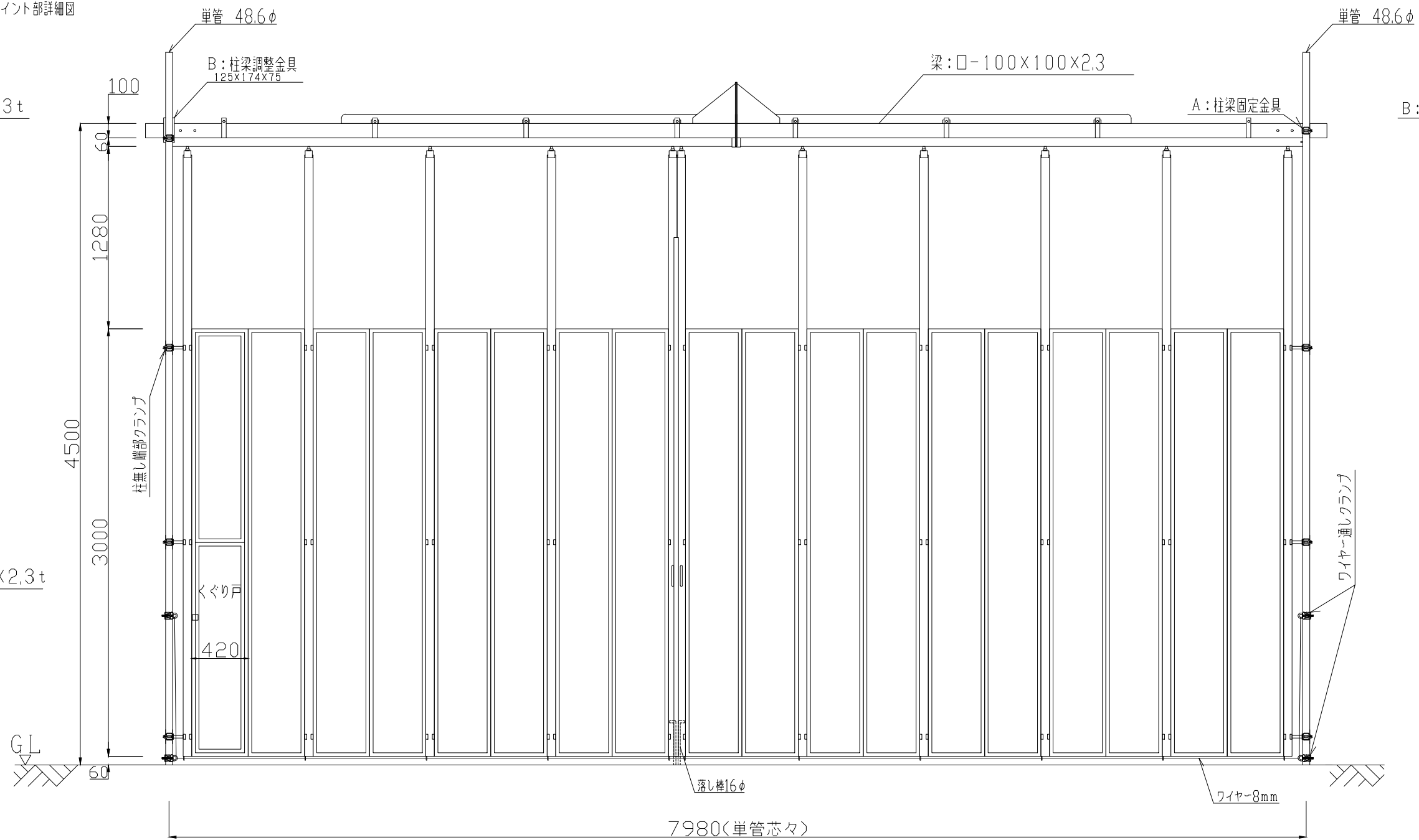
立面图
