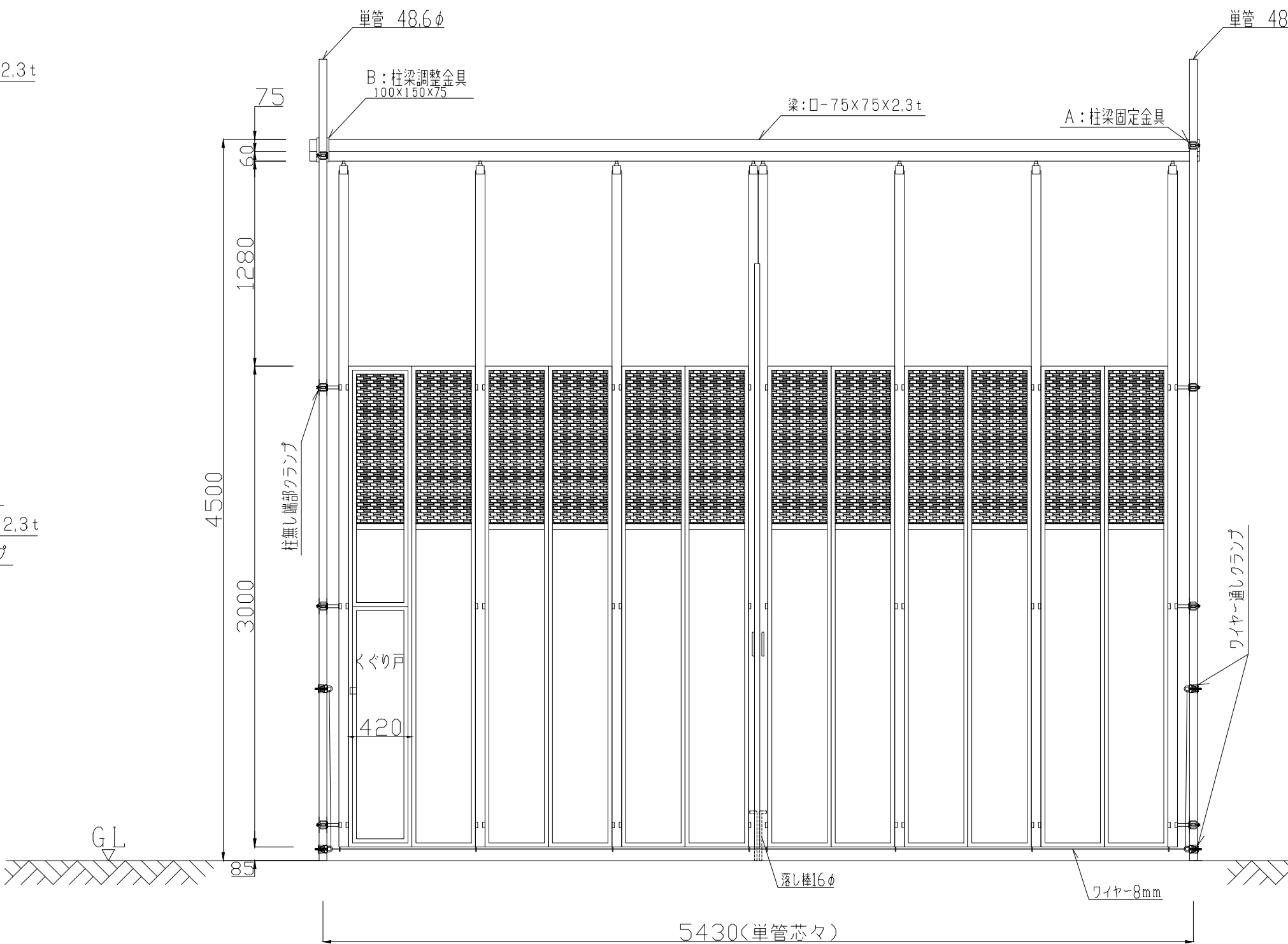
立面図
