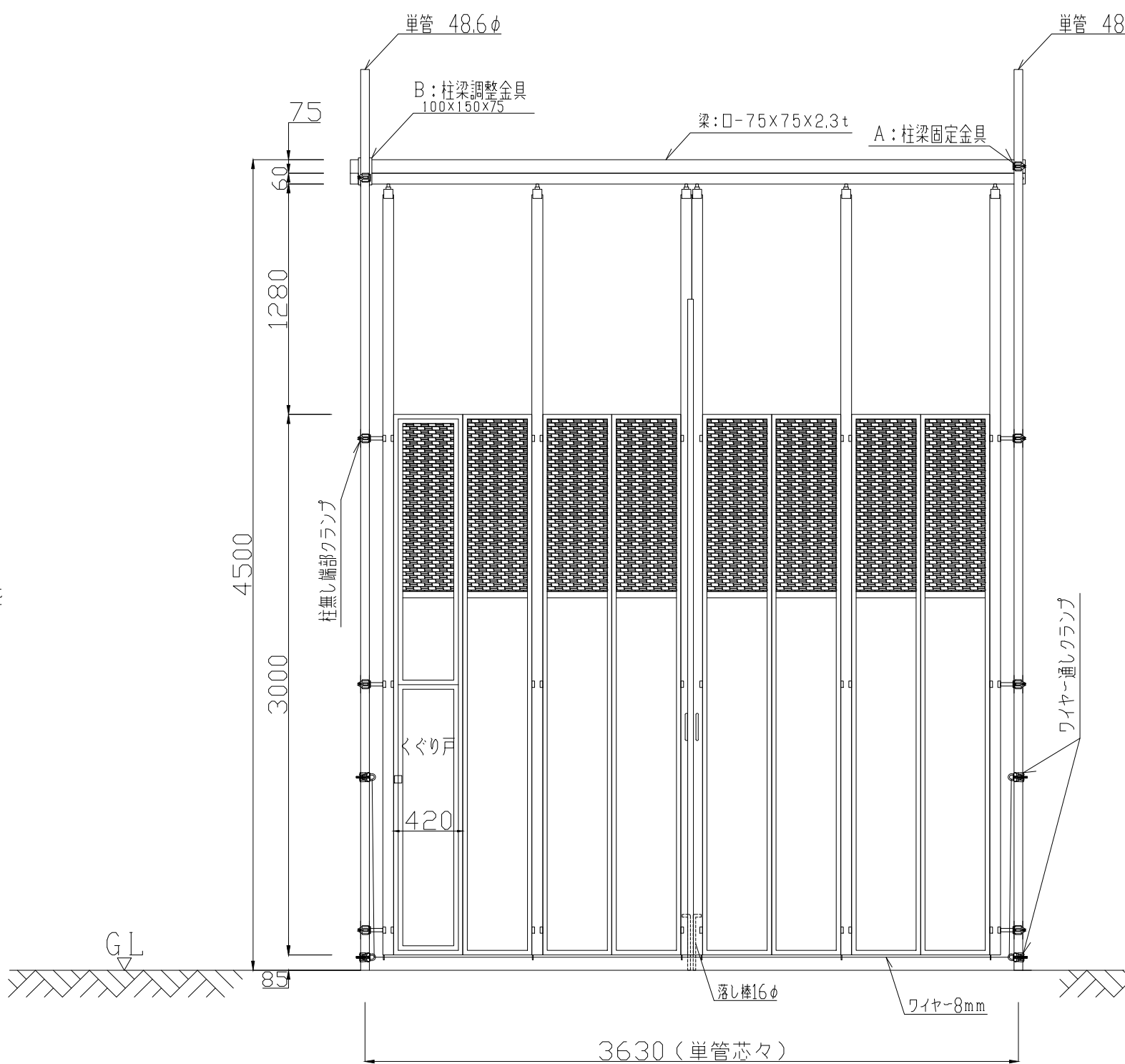
立面図
