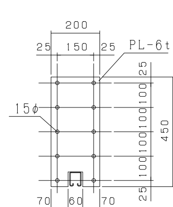
梁ジョイント部詳細図
