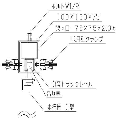
B：柱梁調整金具詳細図
