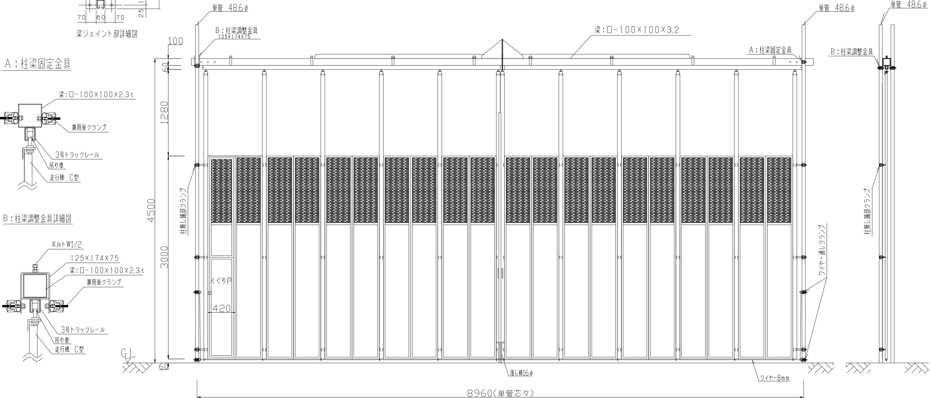
側面図
