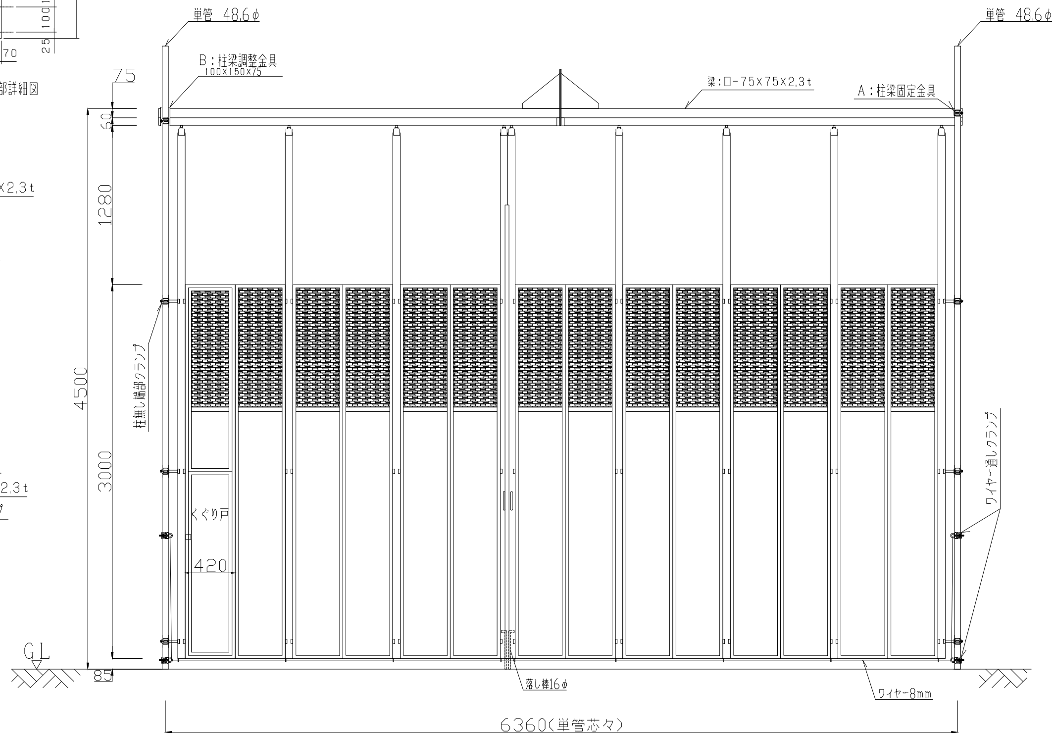
立面图
