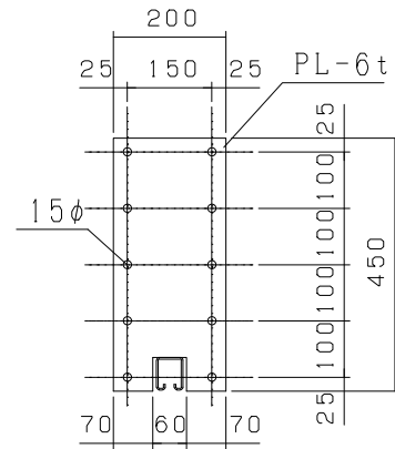
梁ジョイント部詳細図
