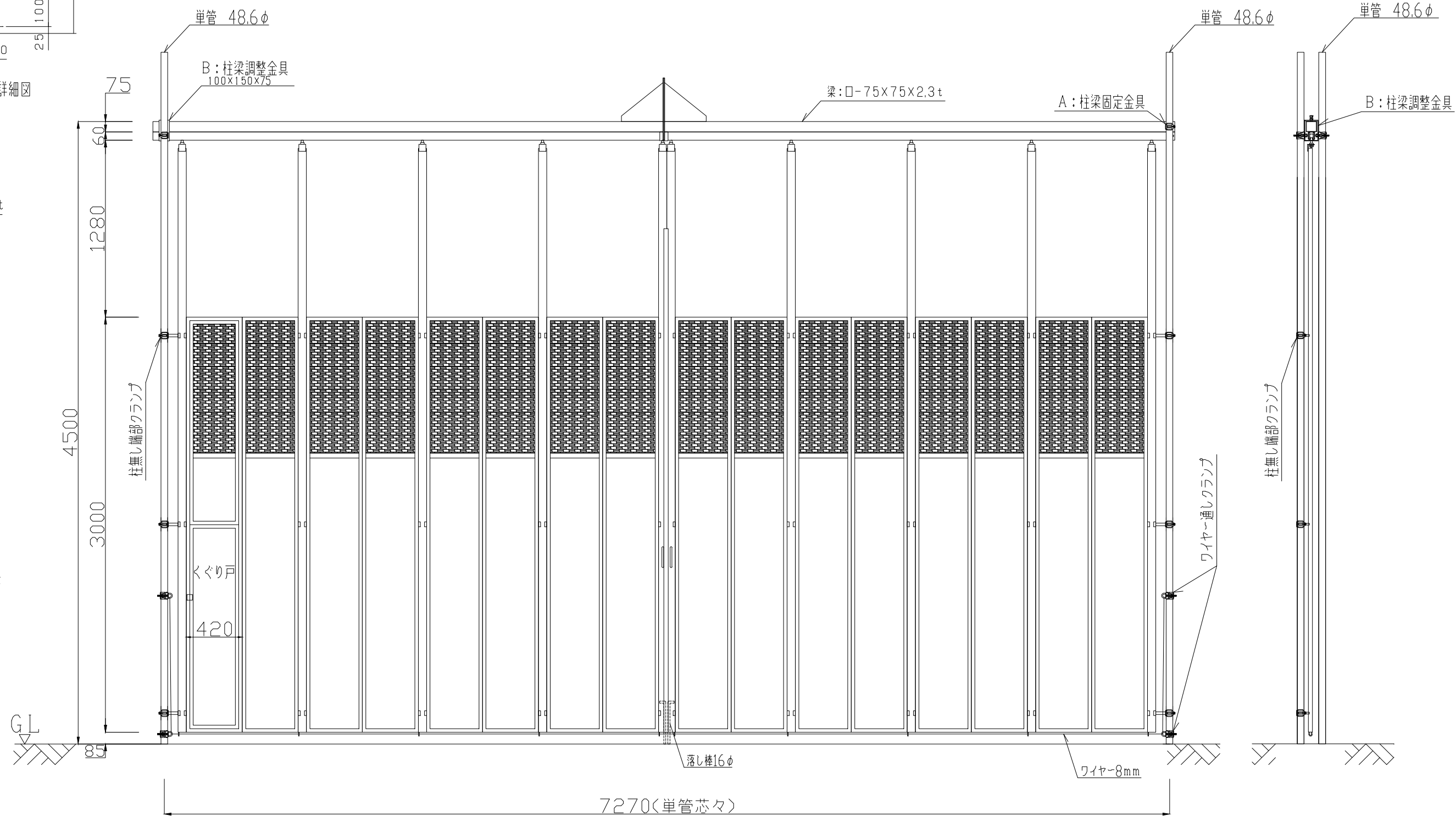
則面义
