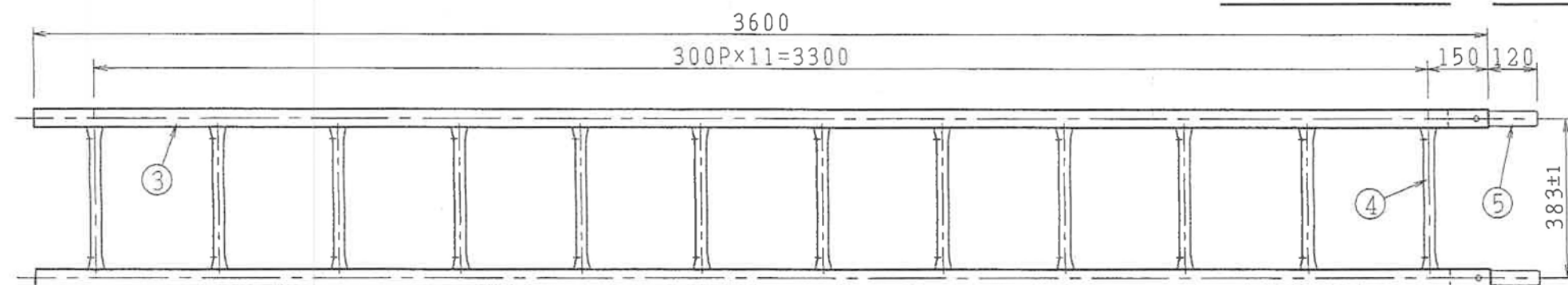
鋼製梯子 3600mm 23Kg
