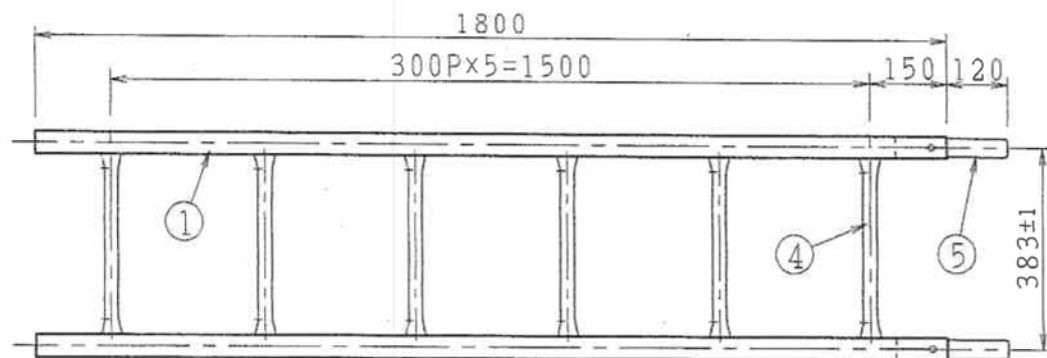
鋼製梯子 1800mm 12Kg
