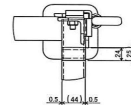
詳細図 a 2ヶ-A (1 : 5)
