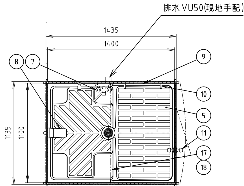
平面
