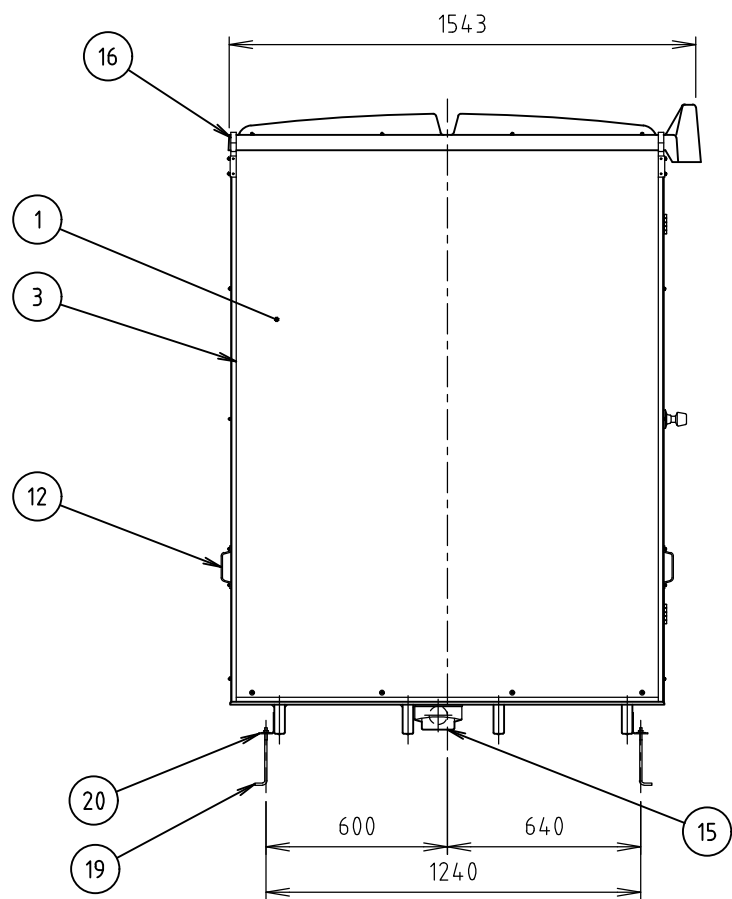
左側面
