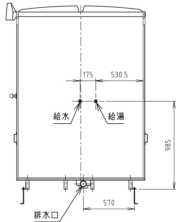
右側面
