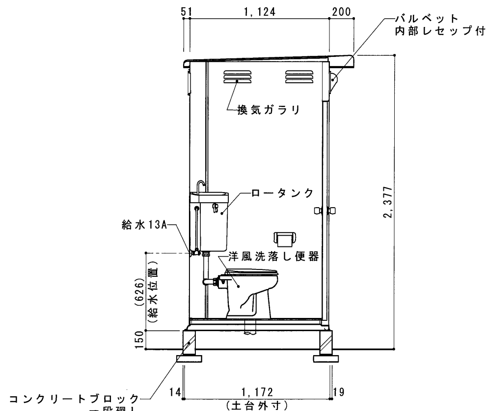
断面図 S=1/30
