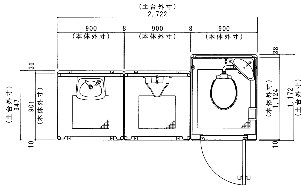
平面図 S=1/30
