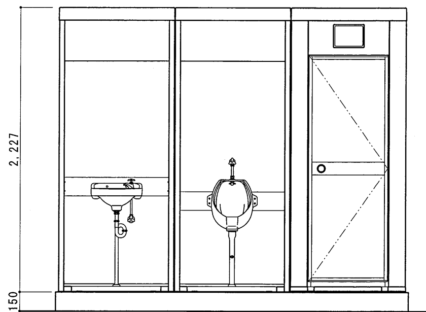
A 立面図 S=1/30
