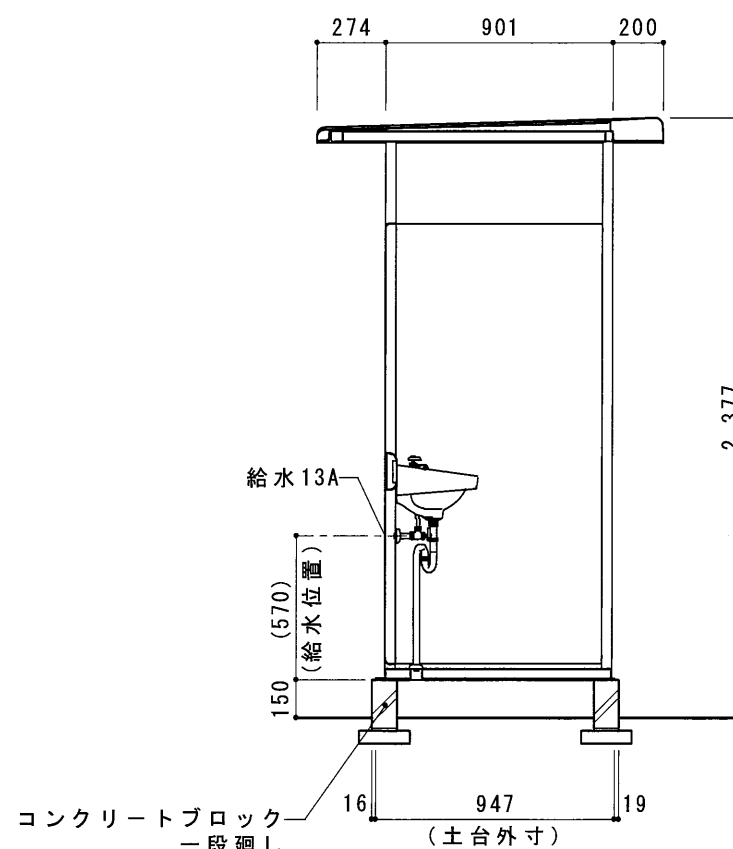
断面図 S=1/30
