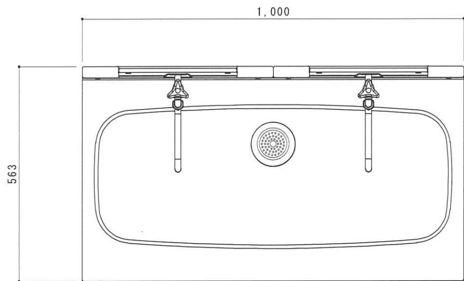
平面図 S=1/10
