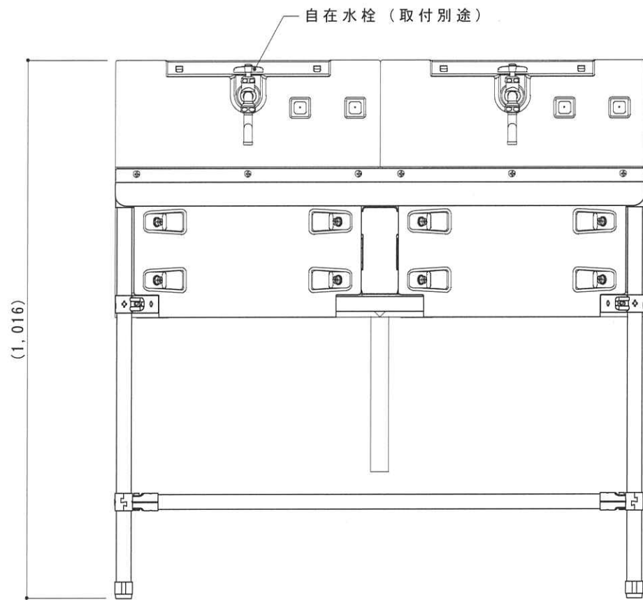
A 立面図 S=1/10
