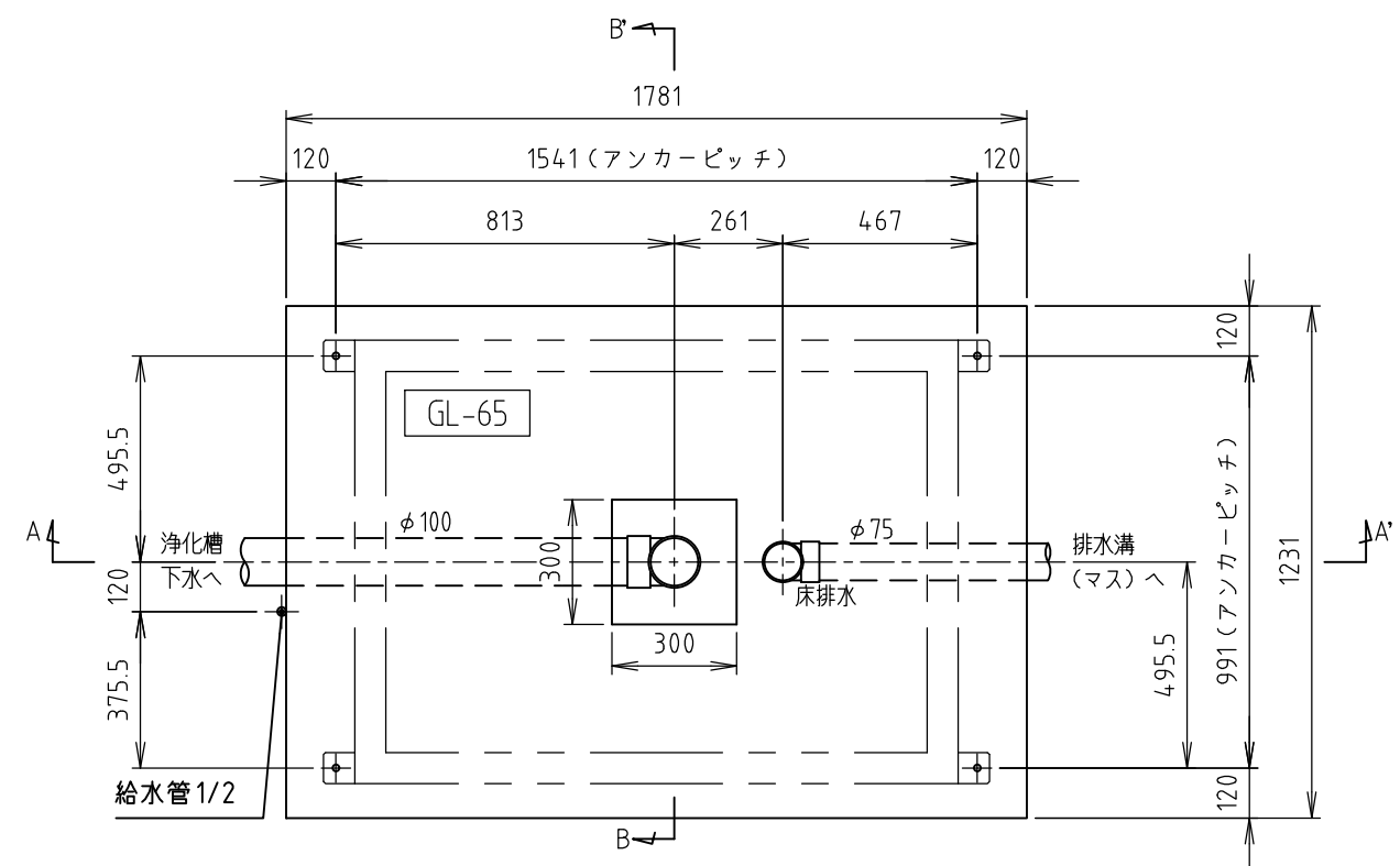
基礎平面図
