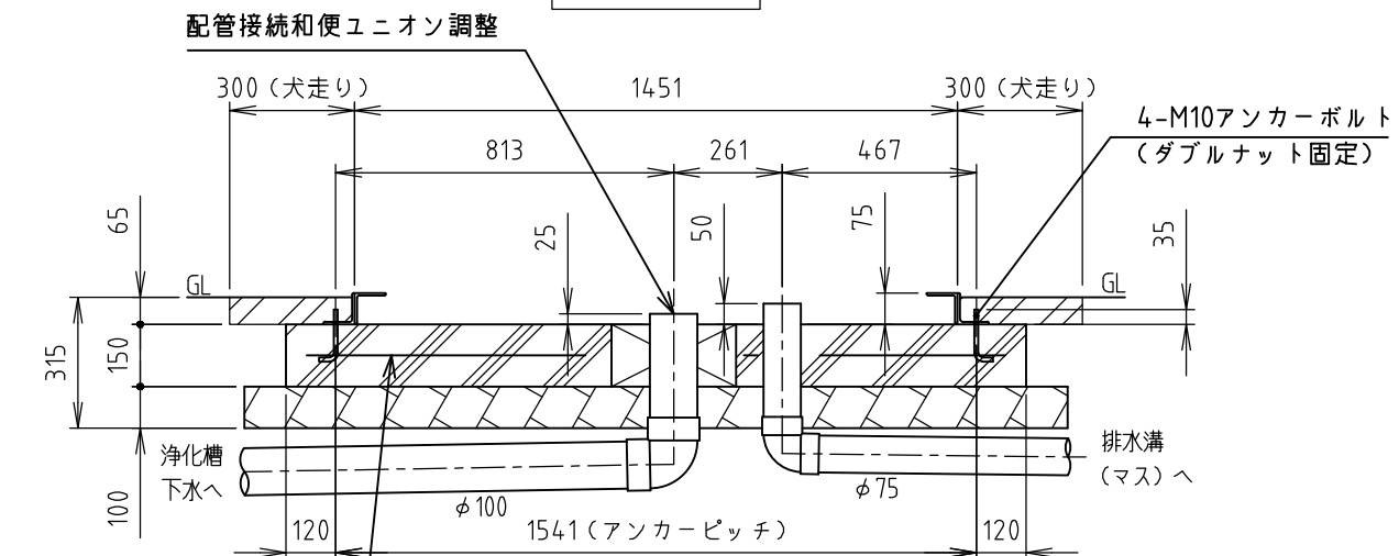
A-A' 断面図
