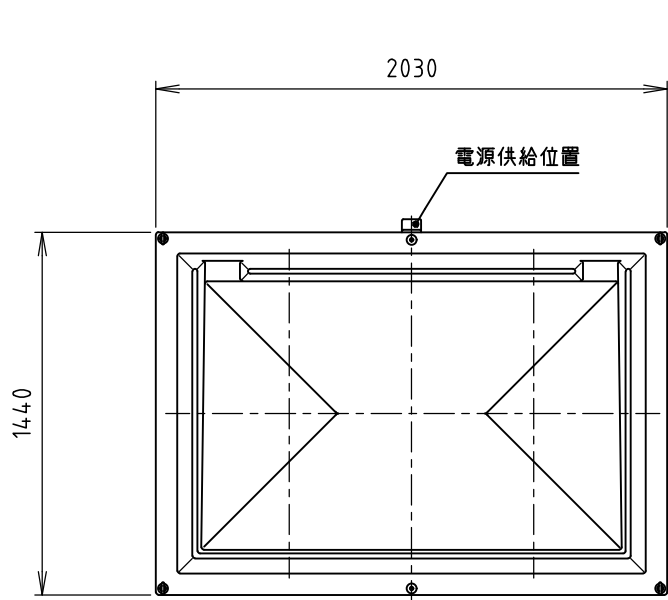
屋根伏図
