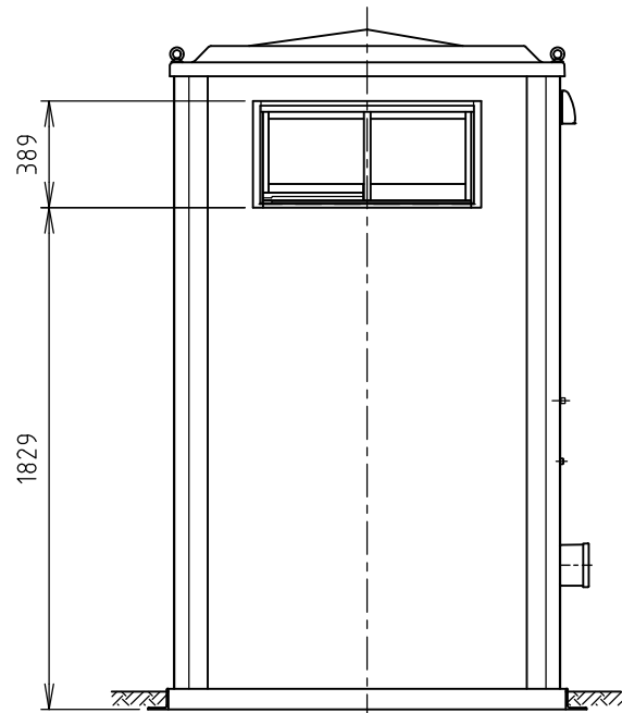
右側面図
