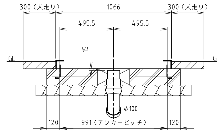
B-B' 断面図
