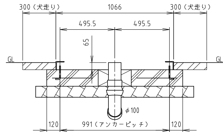
B-B' 断面図
