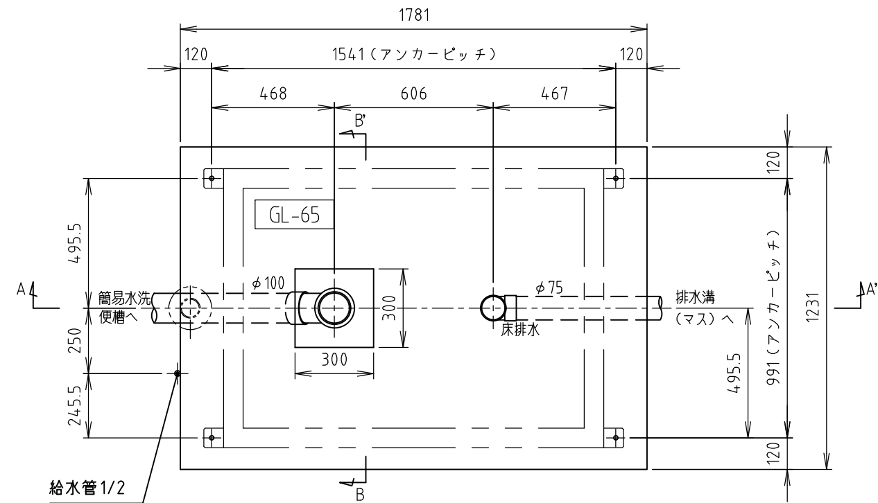
基礎平面図
