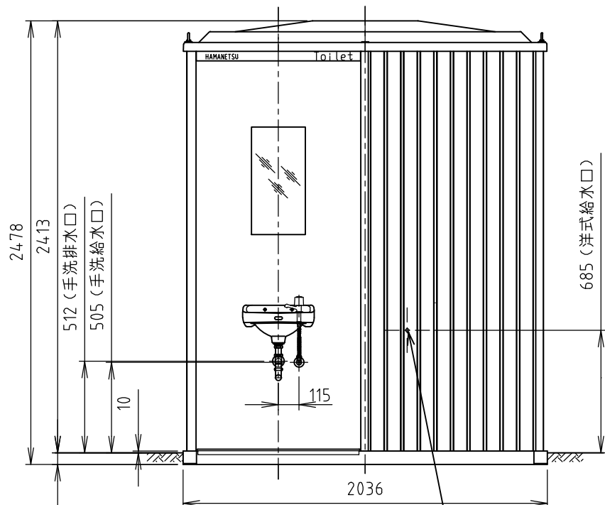
正面図
