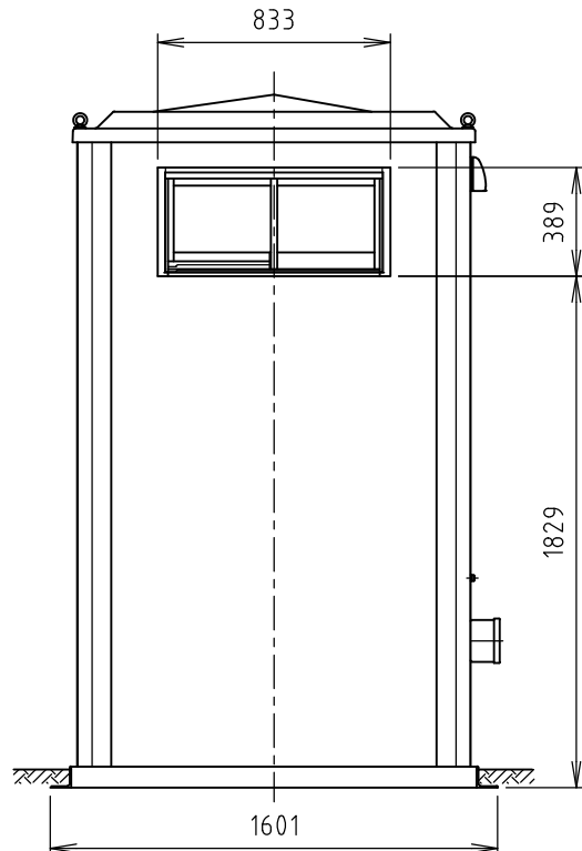
右側面図
