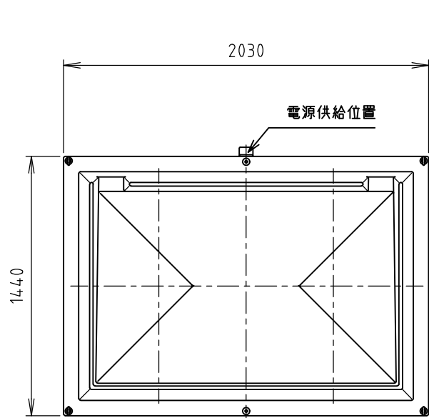
屋根伏図
