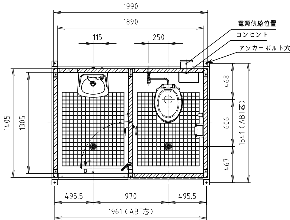
平面図
