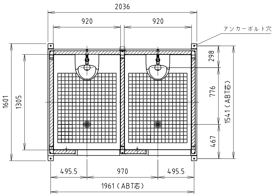
平面図
