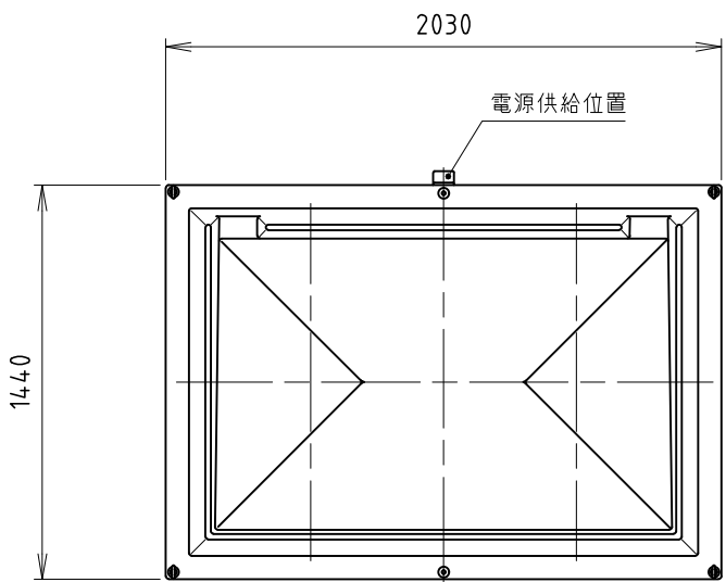
屋根伏図
