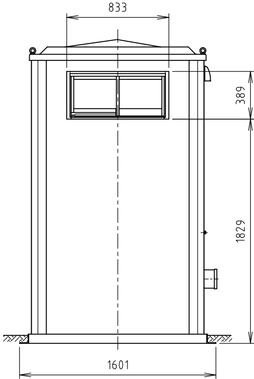
右側面図
