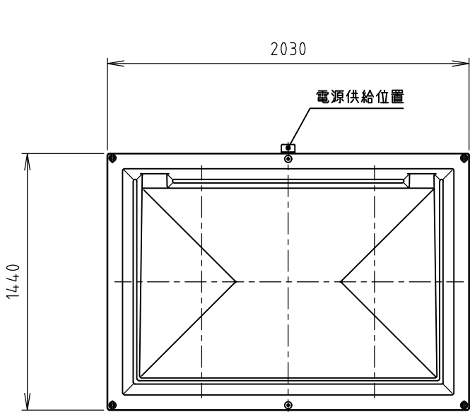
屋根伏図
