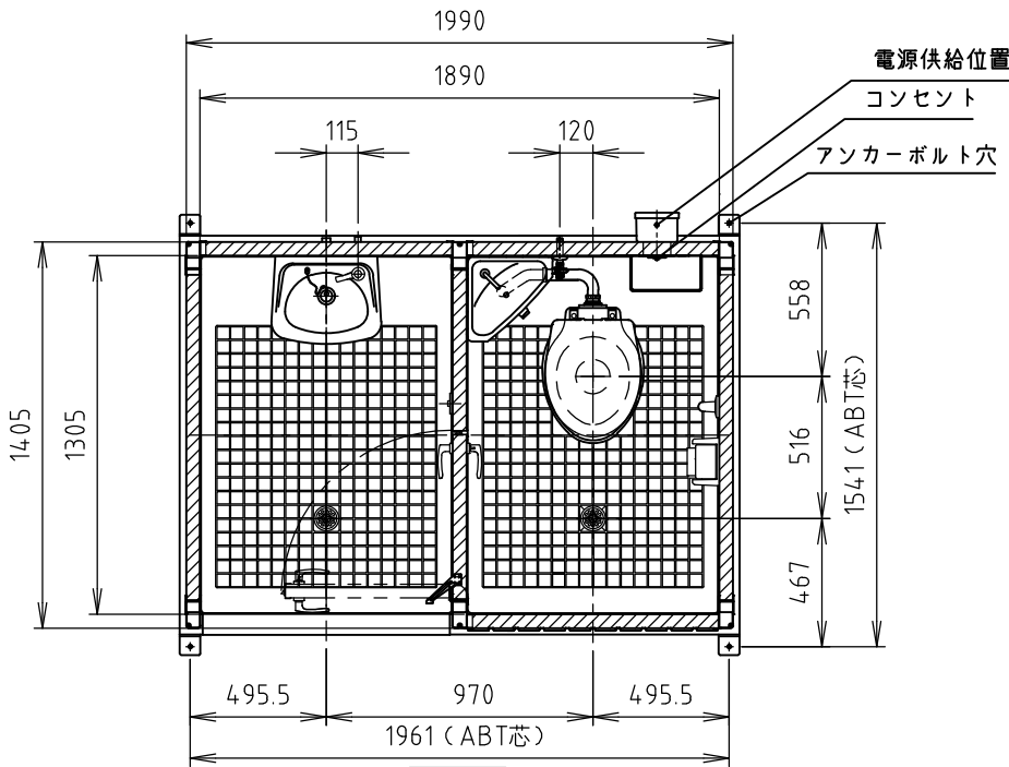
平面図
