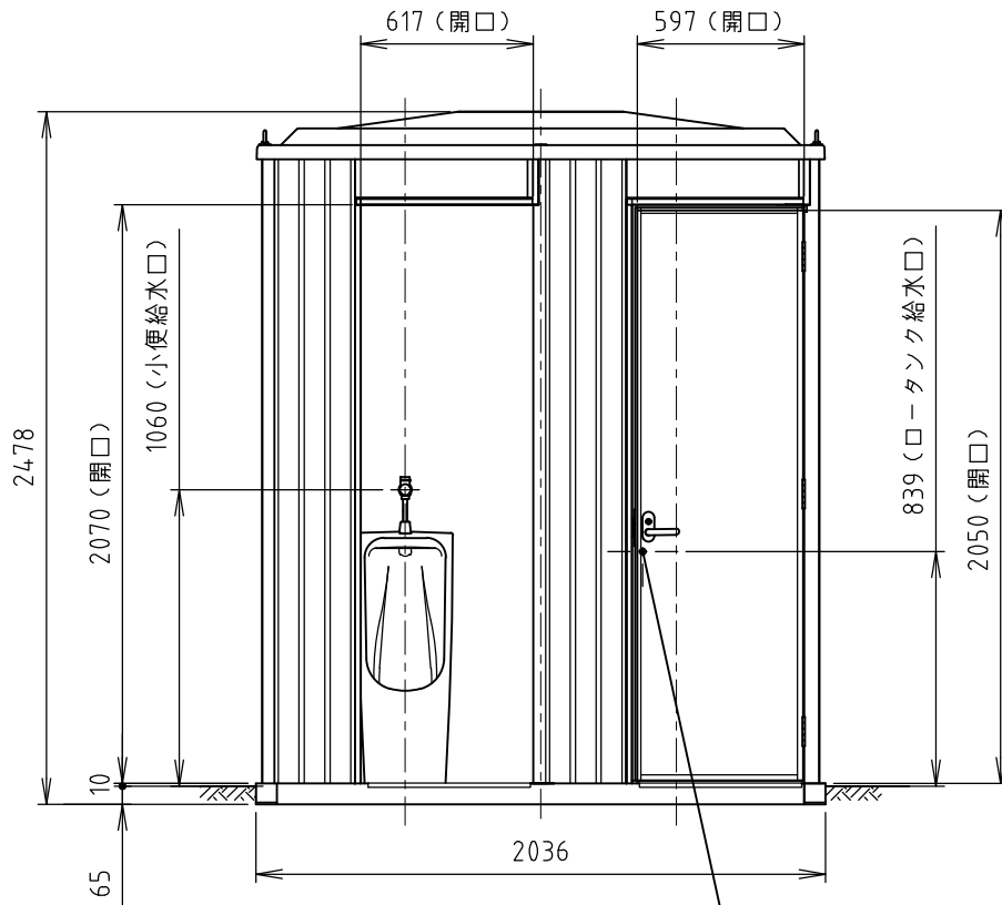
正面図
