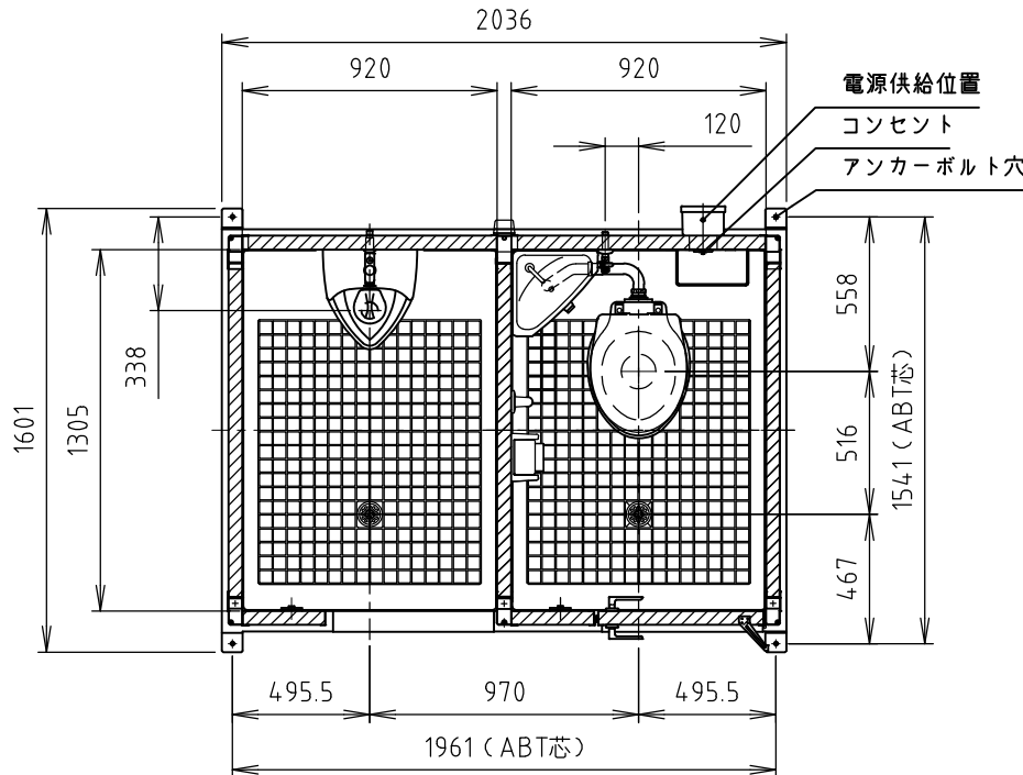
平面図
