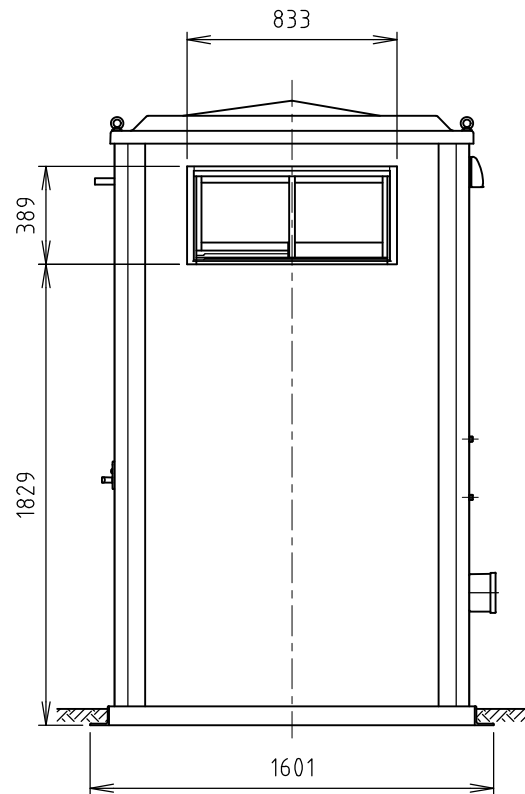
右側面図
