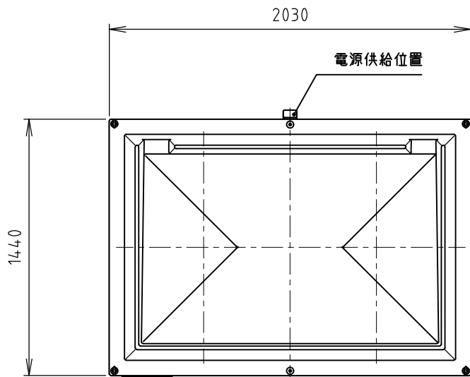
屋根伏図
