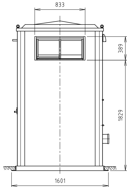
右側面図
