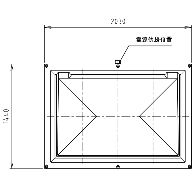
屋根伏図
