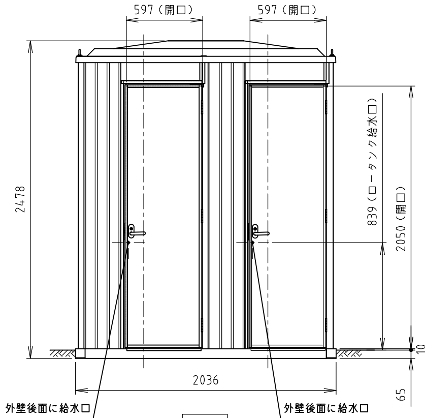
正面図
