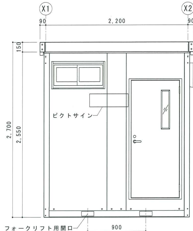
A 立面図 S=1/30
