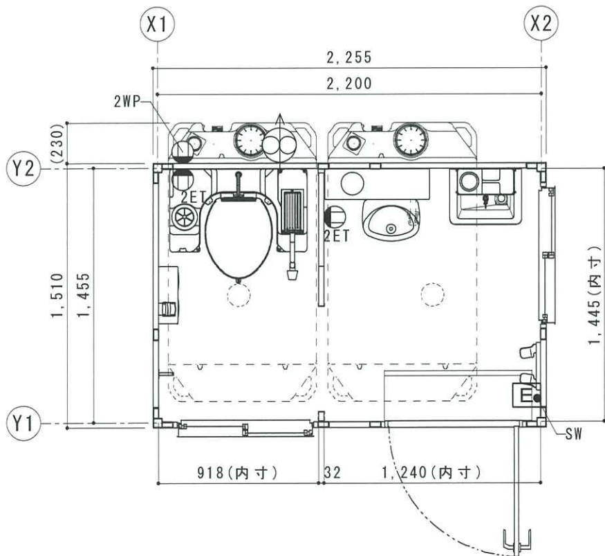
平面図 S=1/30
