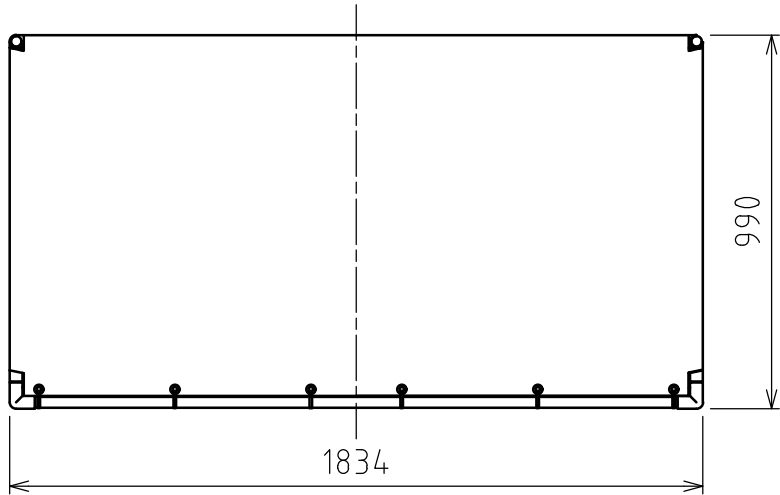
屋根伏図
