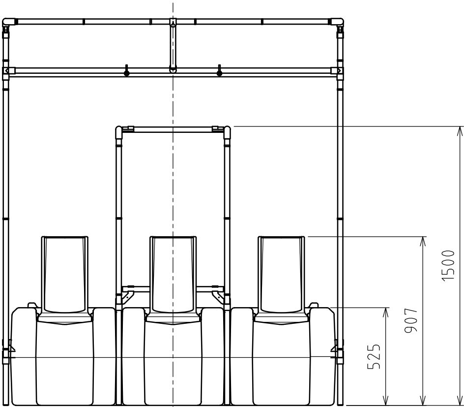
正面図
