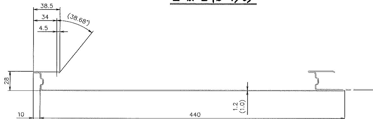
断面詳細図 (S=1/1)
