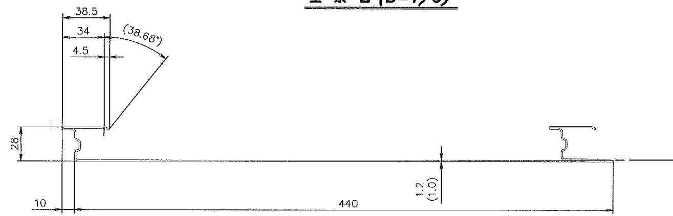
断面詳細図 (S=1/1)
