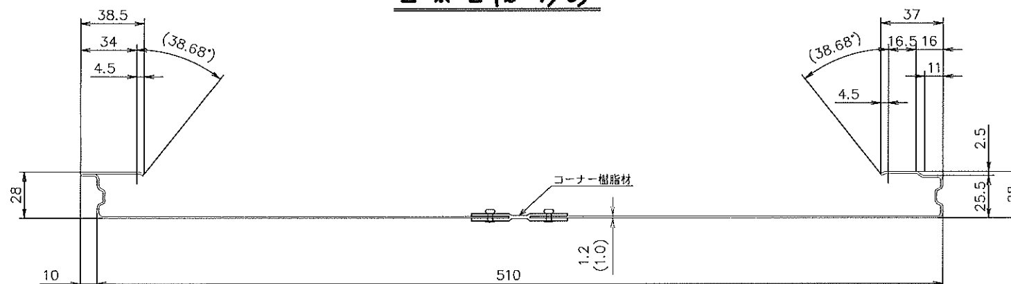
標準仕様
